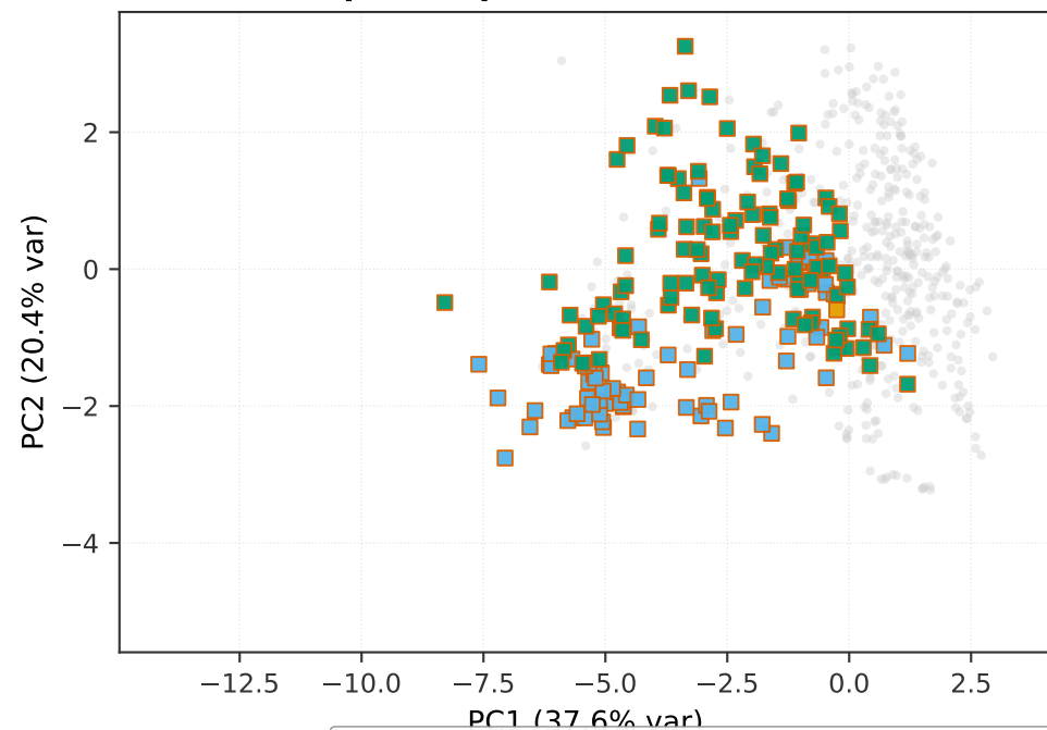
(c) ArcPL · Opx + Liquid
