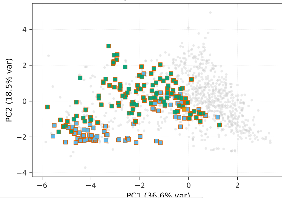
(d) ArcPL · Opx only
