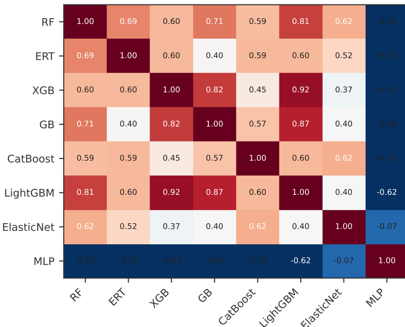
(a) Opx + Liquid · T (°C) med \rho=0.58
