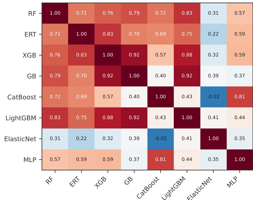
(b) Opx + Liquid · P (kbar) med \rho=0.59
