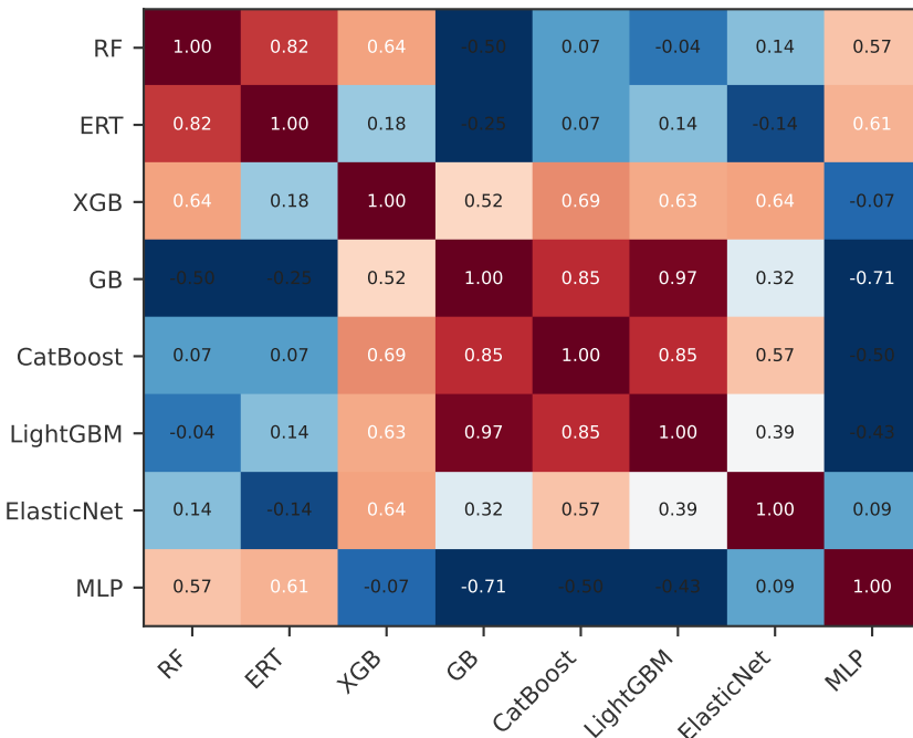
(c) Opx only · T (°C) med \rho=0.25
