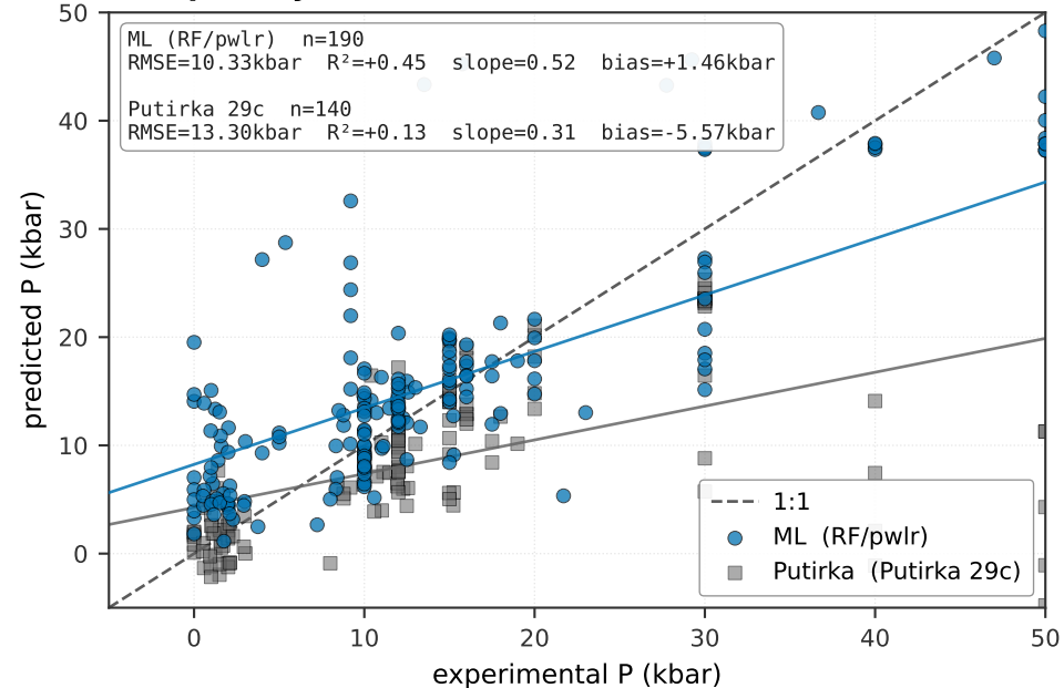
(d) opx-only · P (kbar)
