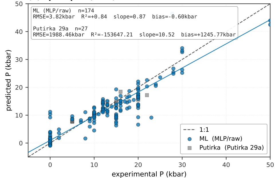
(b) opx-liq · P (kbar)
