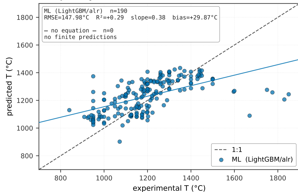
(c) opx-only · T (°C)
