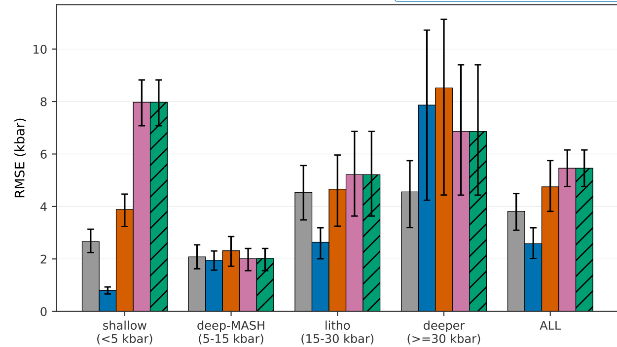
(b) Opx + Liquid P (kbar)
