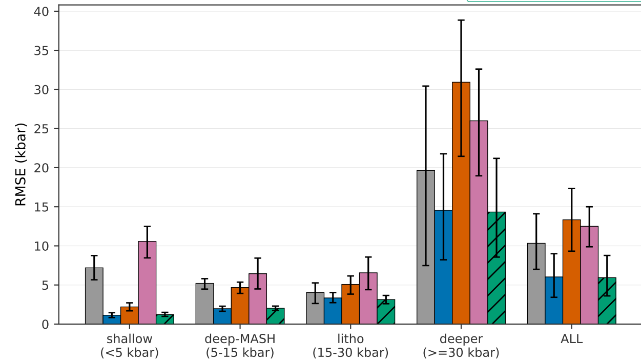
(d) Opx only P (kbar)
