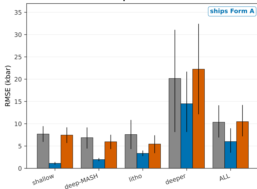
(d) Opx only P (kbar) corrected model: RF + pwlr
