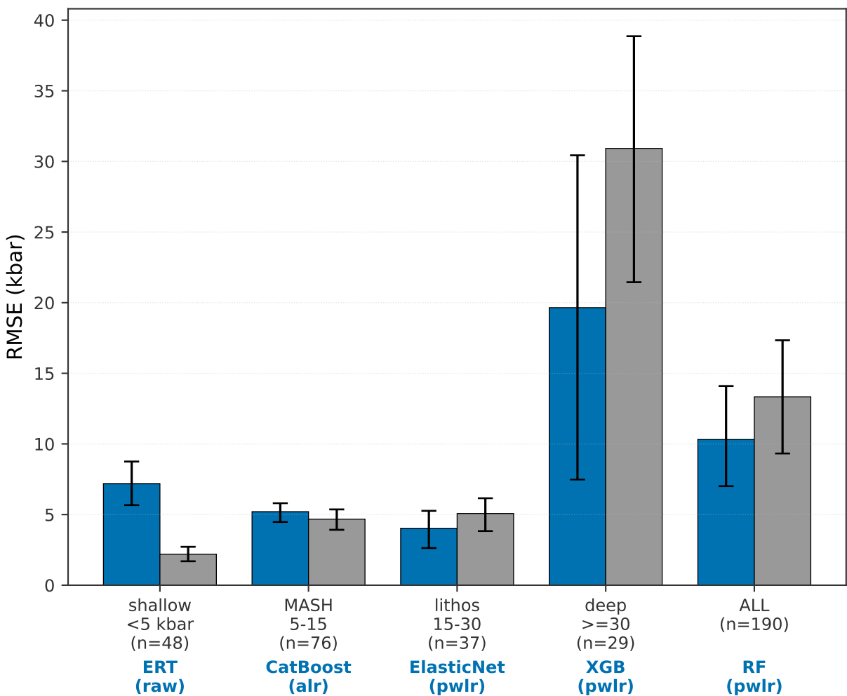
(d) Opx only P (kbar)
