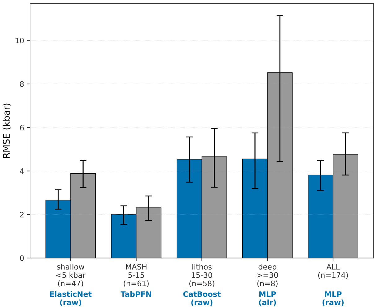
(b) Opx + Liquid P (kbar)
