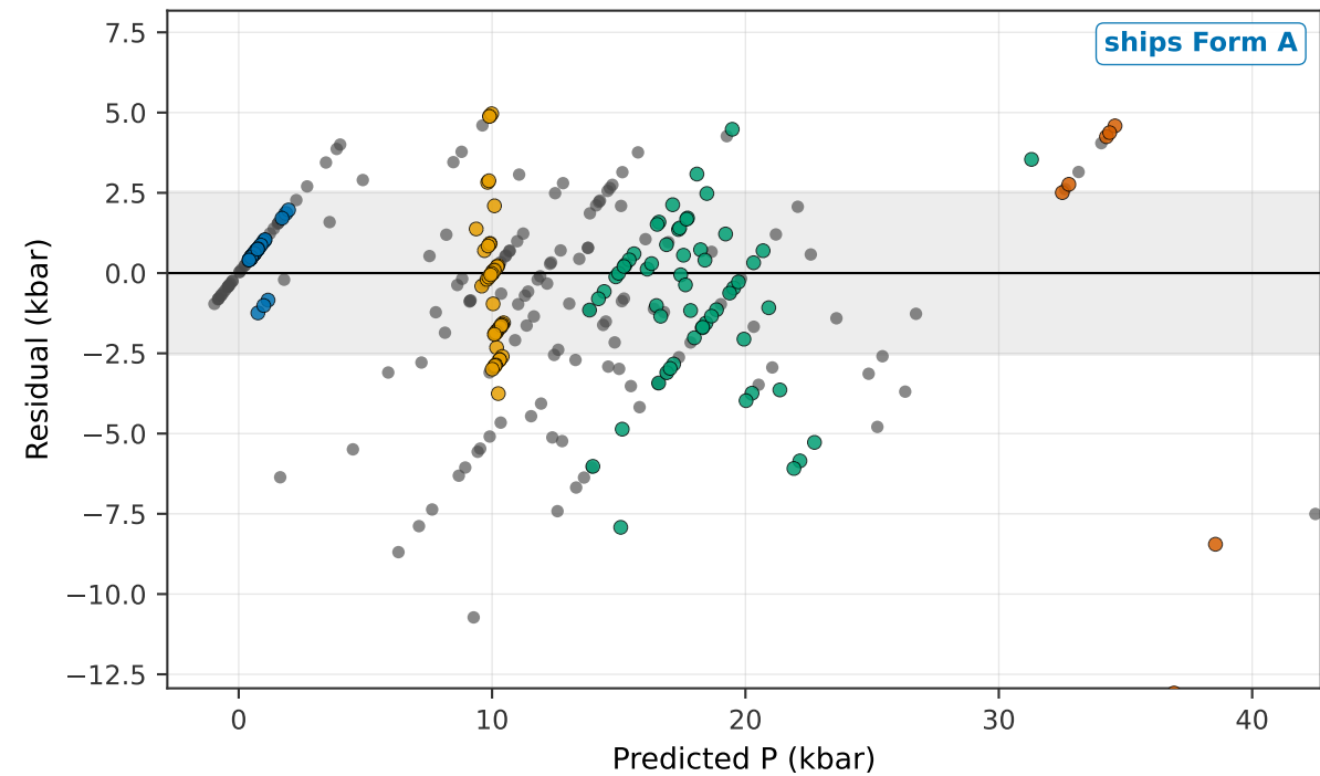
(d) Opx only P (kbar) corrected model: RF + pwlr
