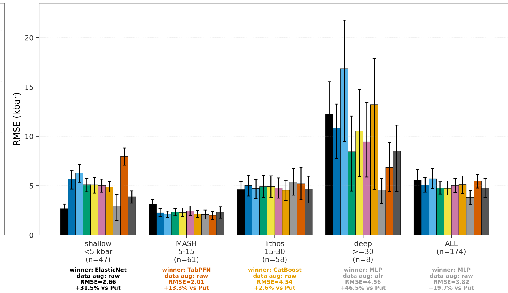
(b) Opx + Liquid P (kbar)
