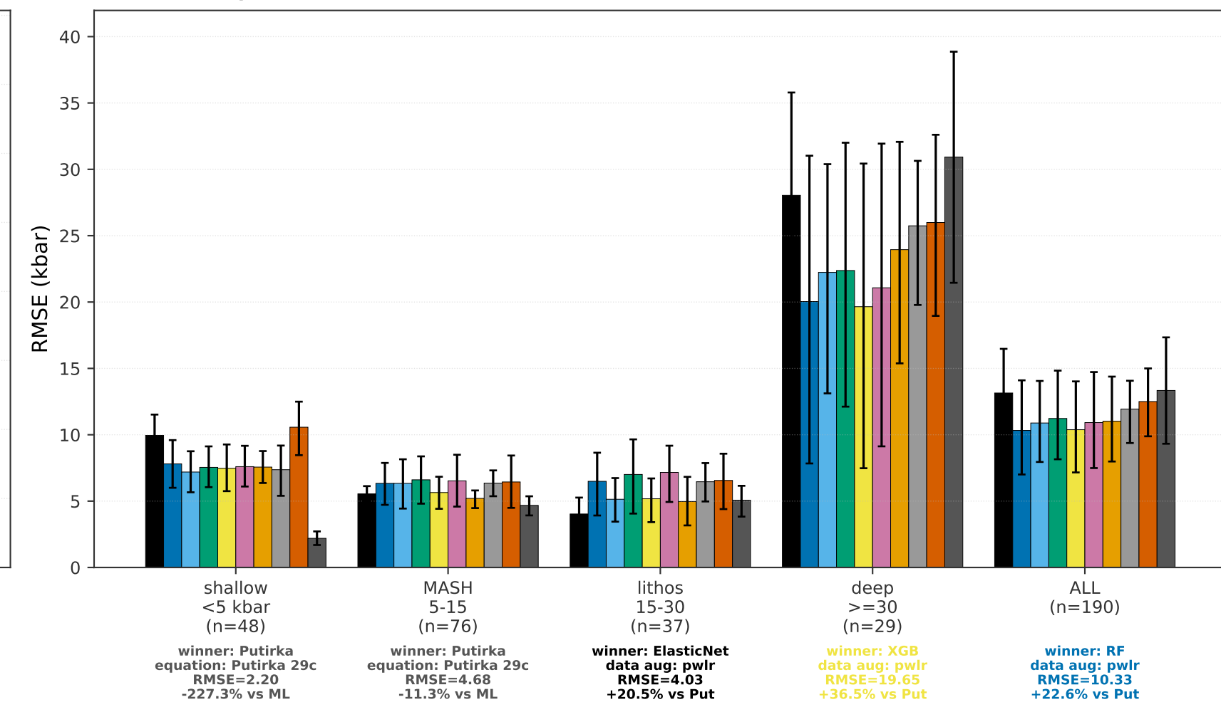
(d) Opx only P (kbar)
