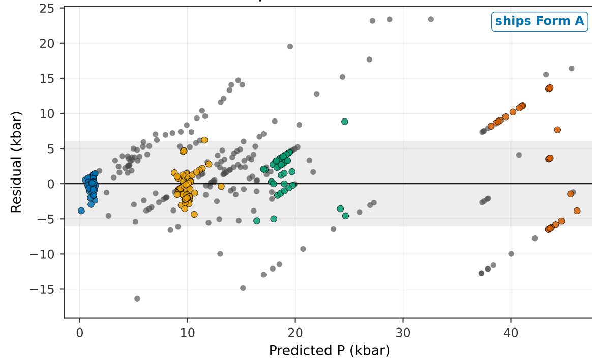
(d) Opx only P (kbar) corrected model: RF + pwlr
