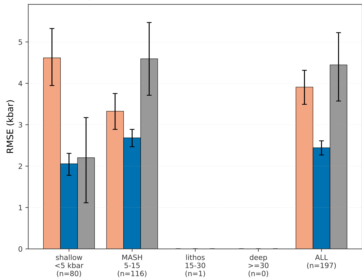
(d) Opx only P (kbar)
