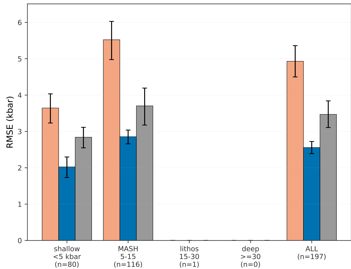
(b) Opx + Liquid P (kbar)
