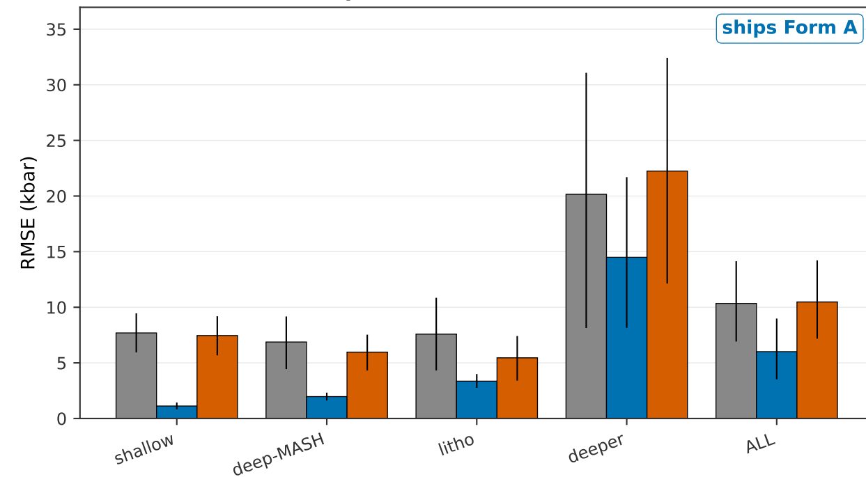
(d) Opx only P (kbar) corrected model: RF + pwlr
