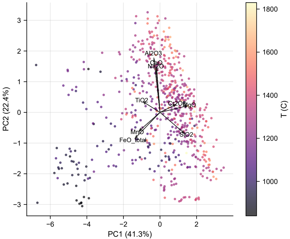
opx PCA biplot
