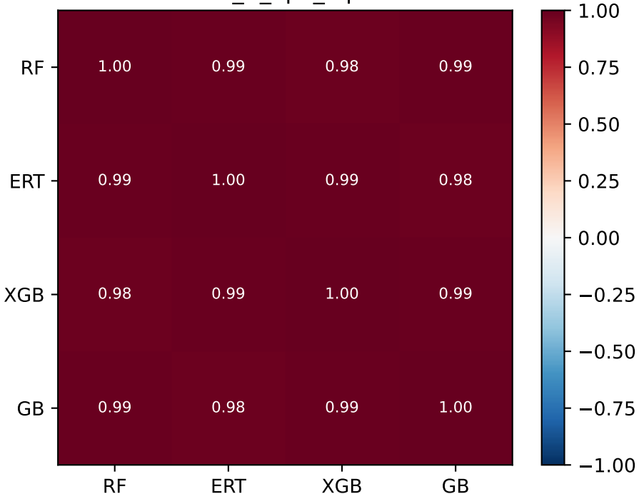
T_C_opx_only
