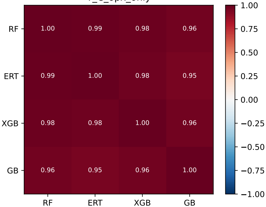
T_C_opx_only
