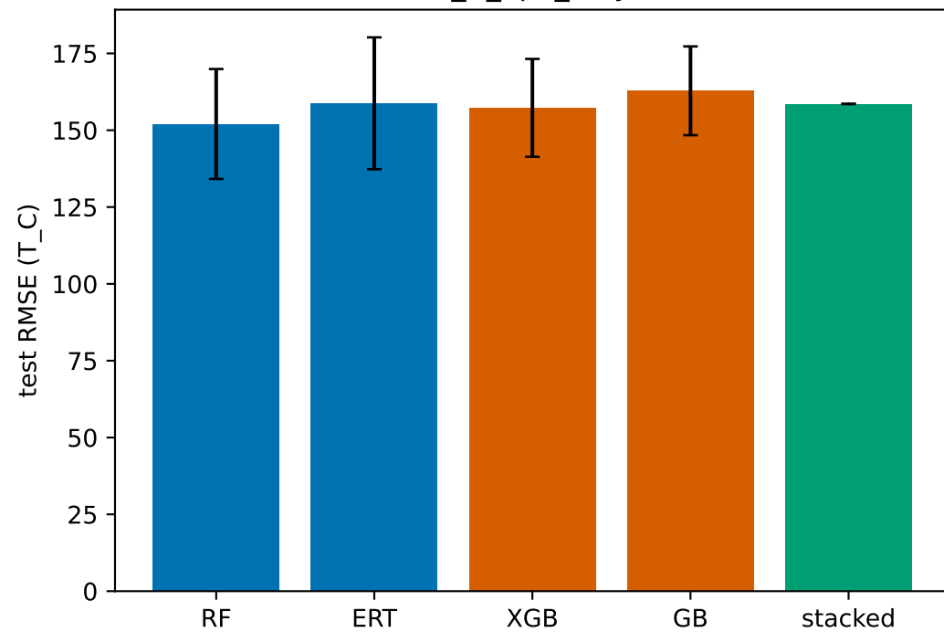
T_C_opx_only
