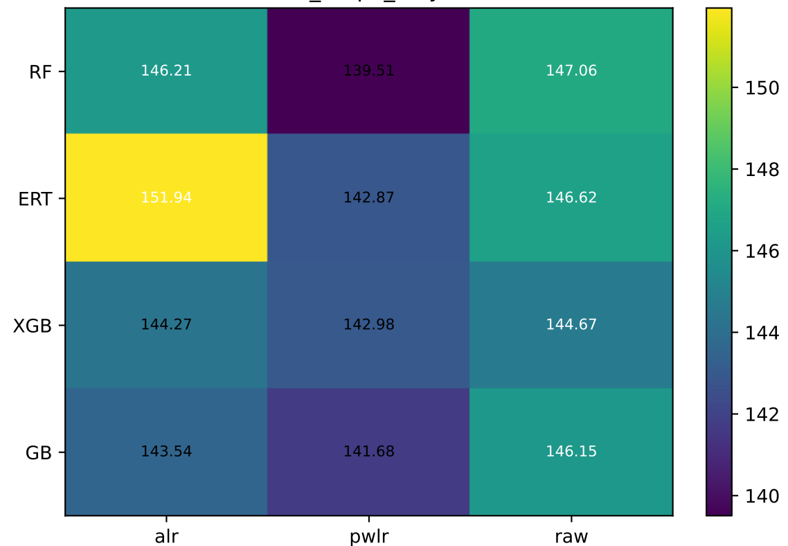
P_kbar opx_only
