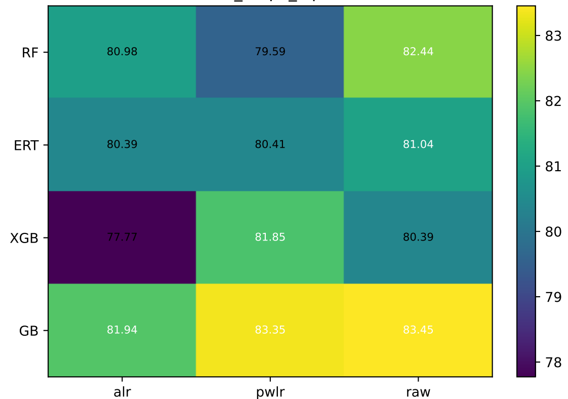
P_kbar opx_liq
