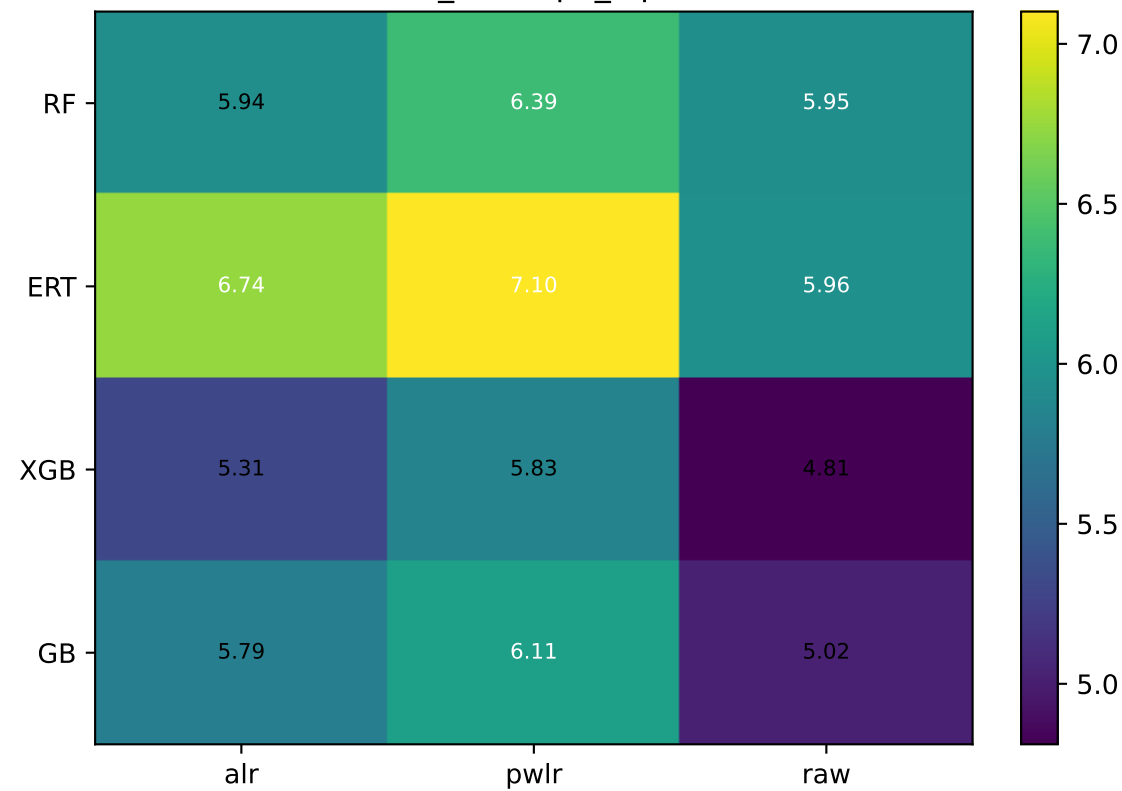
P_kbar opx_liq
