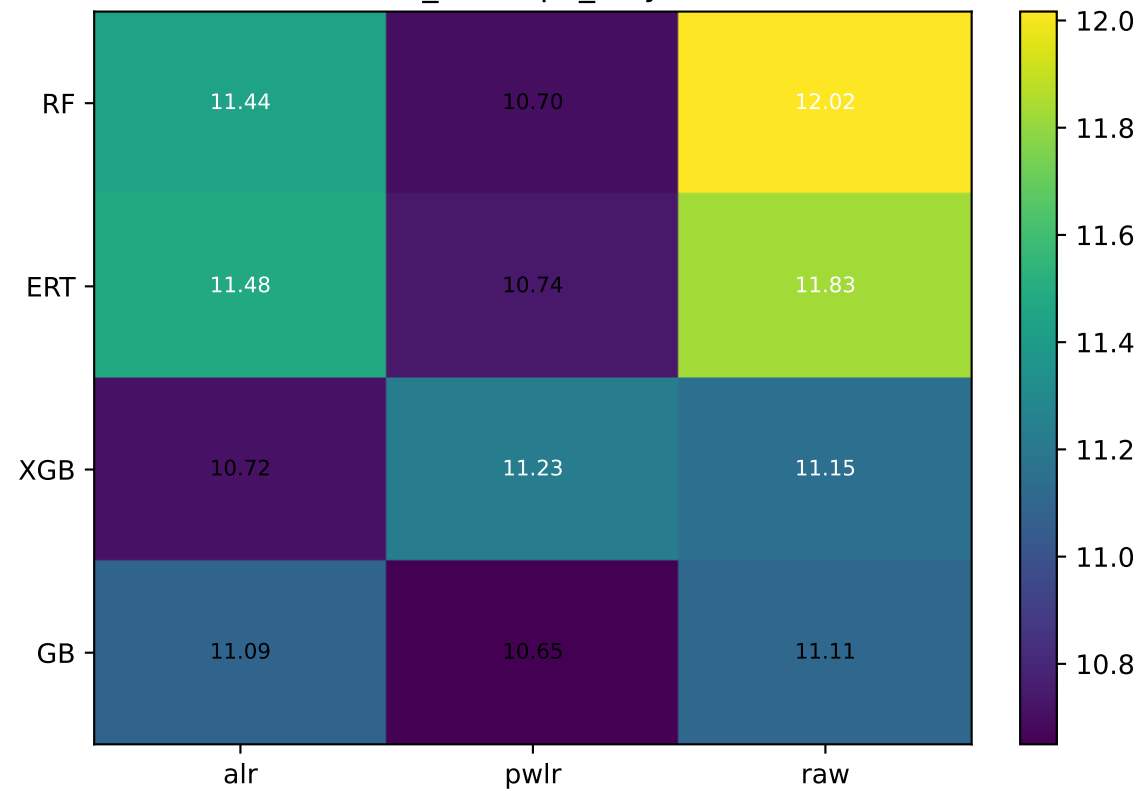
P_kbar opx_only
