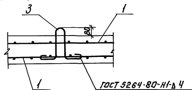
Деталь установки монтажной петли.
