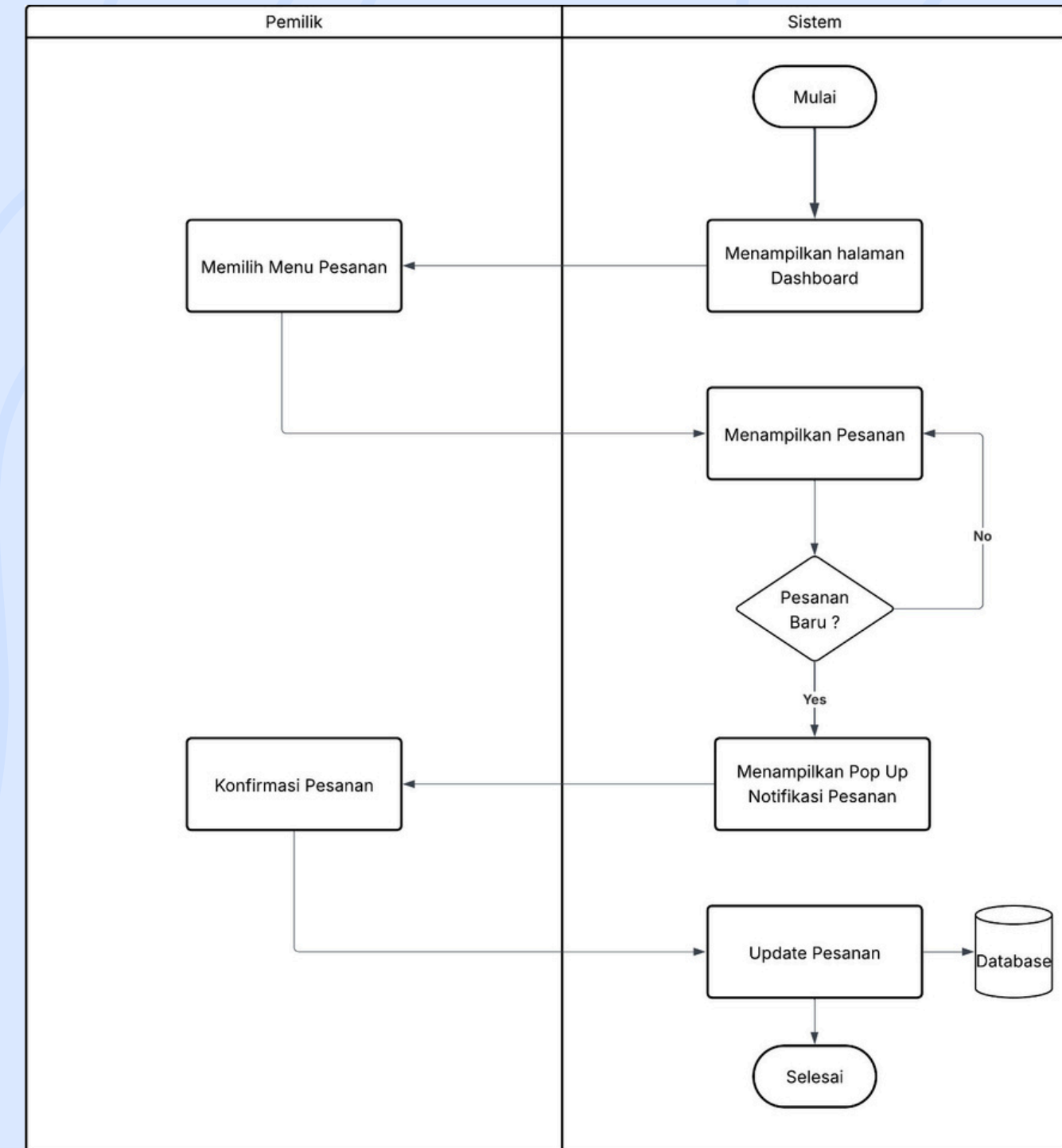
Proses Pengolaan
