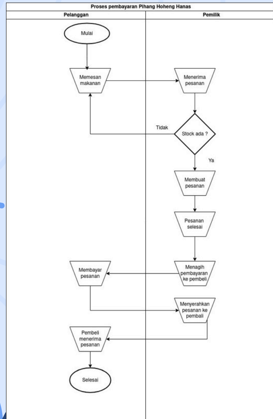
Proses pembayaran
