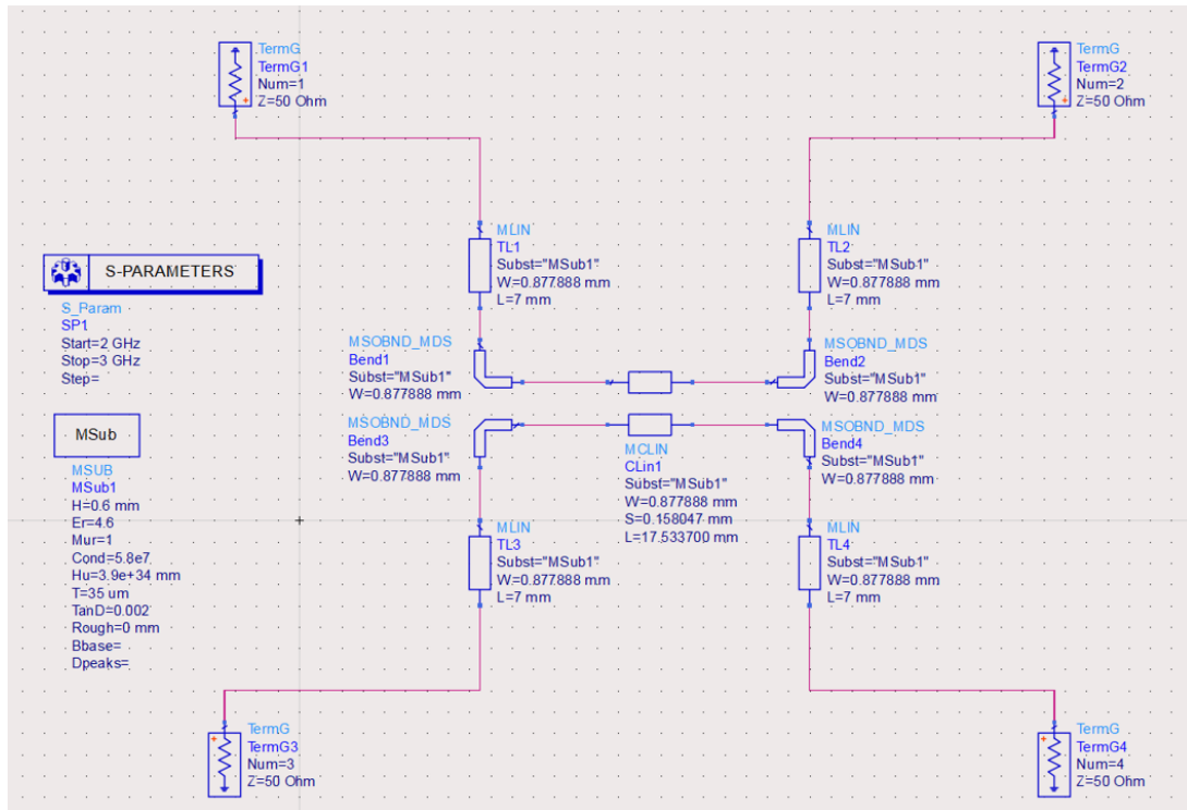
Hình 3.13: Schematic sau khi đã nhập thông số kích thước của microstrip.
