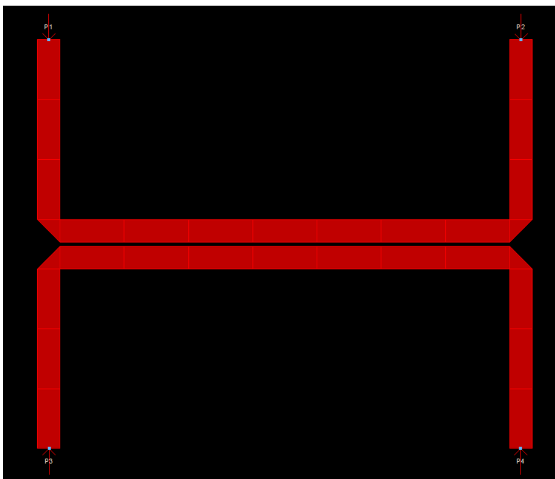
Hình 3.15: Layout của Coupled Line Directional Coupler.
