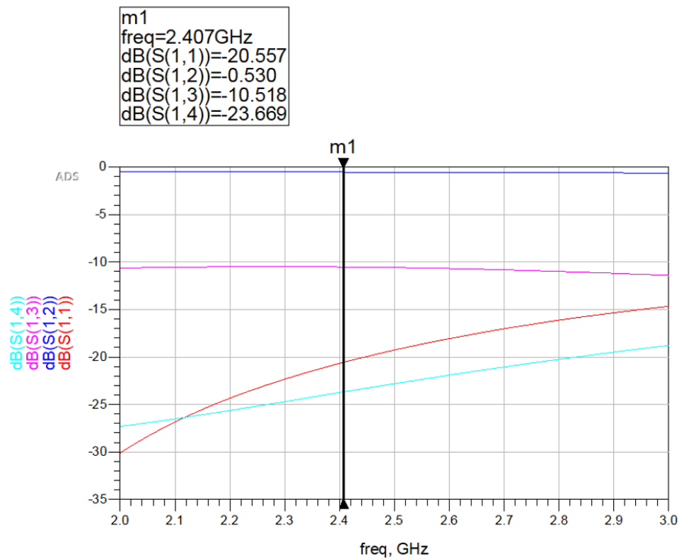
Hình 3.14: Kết quả mô phỏng.
