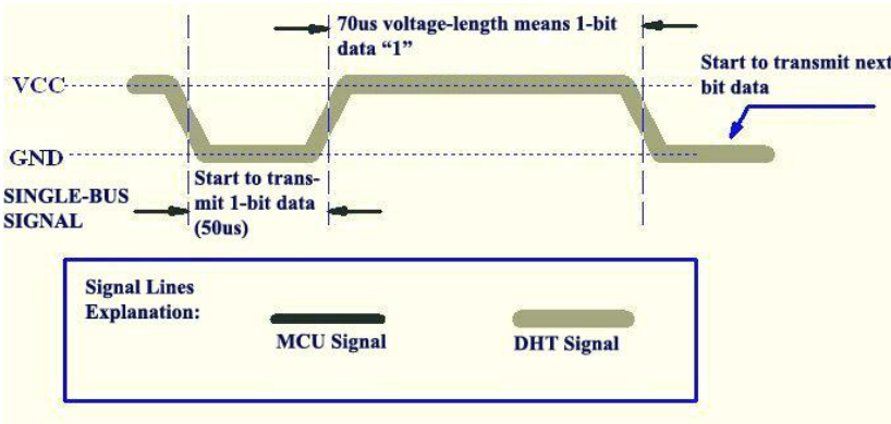
Hình 3.4: Data "1" indication.
