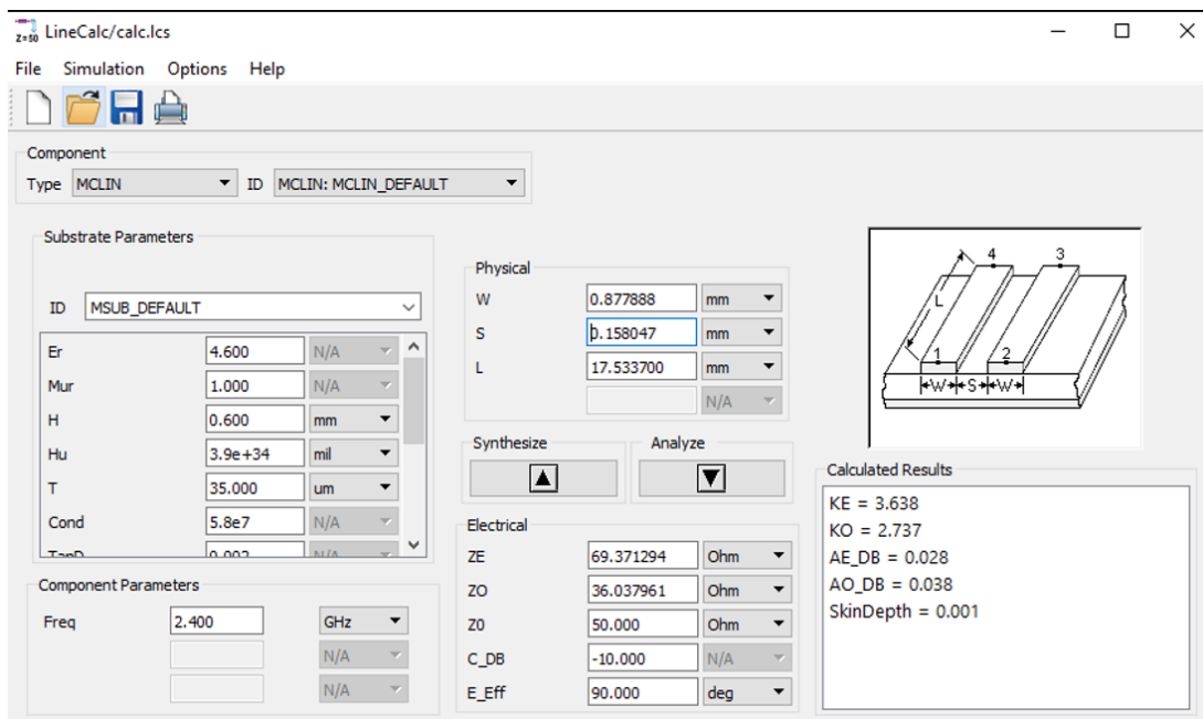
Hình 3.12: Các thông số kích thước đường dây sau khi chạy công cụ LineCalc.
