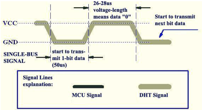
Hình 3.3: Data "0" indication.
