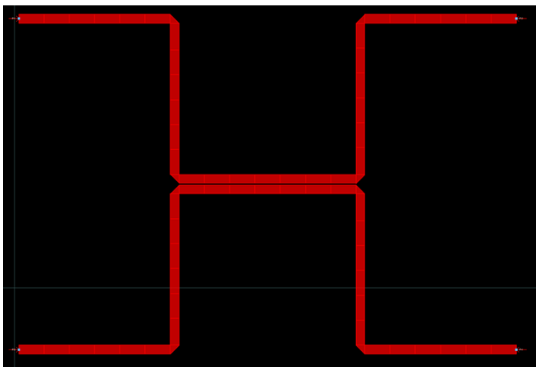
Hình 3.15: Layout của Coupled Line Directional Coupler.
