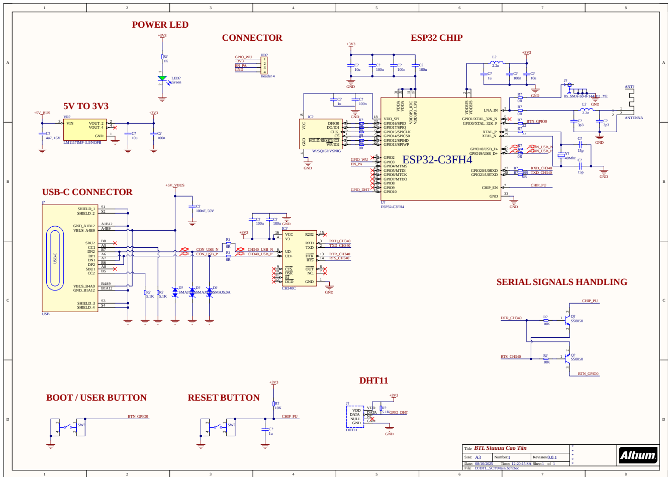
Hình 3.5: Schematic of a BLE node using ESP32-C3.
