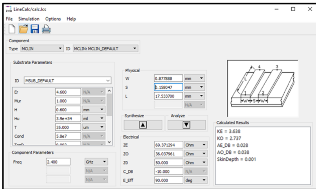
Hình 3.11: Các thông số kích thước đường dây sau khi chạy công cụ LineCalc.
