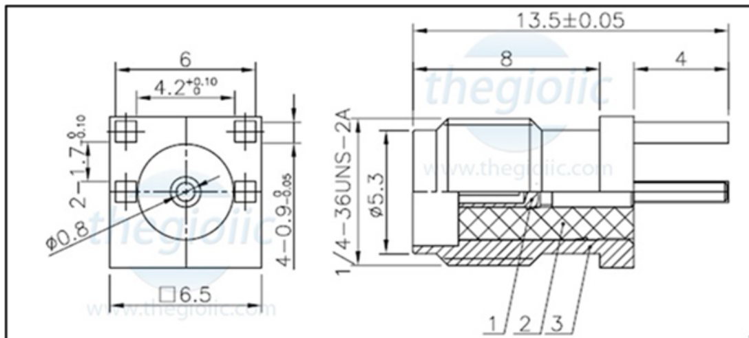
Hình 3.12: Các thông số kích thước của đầu SMA cái 13.5mm.
