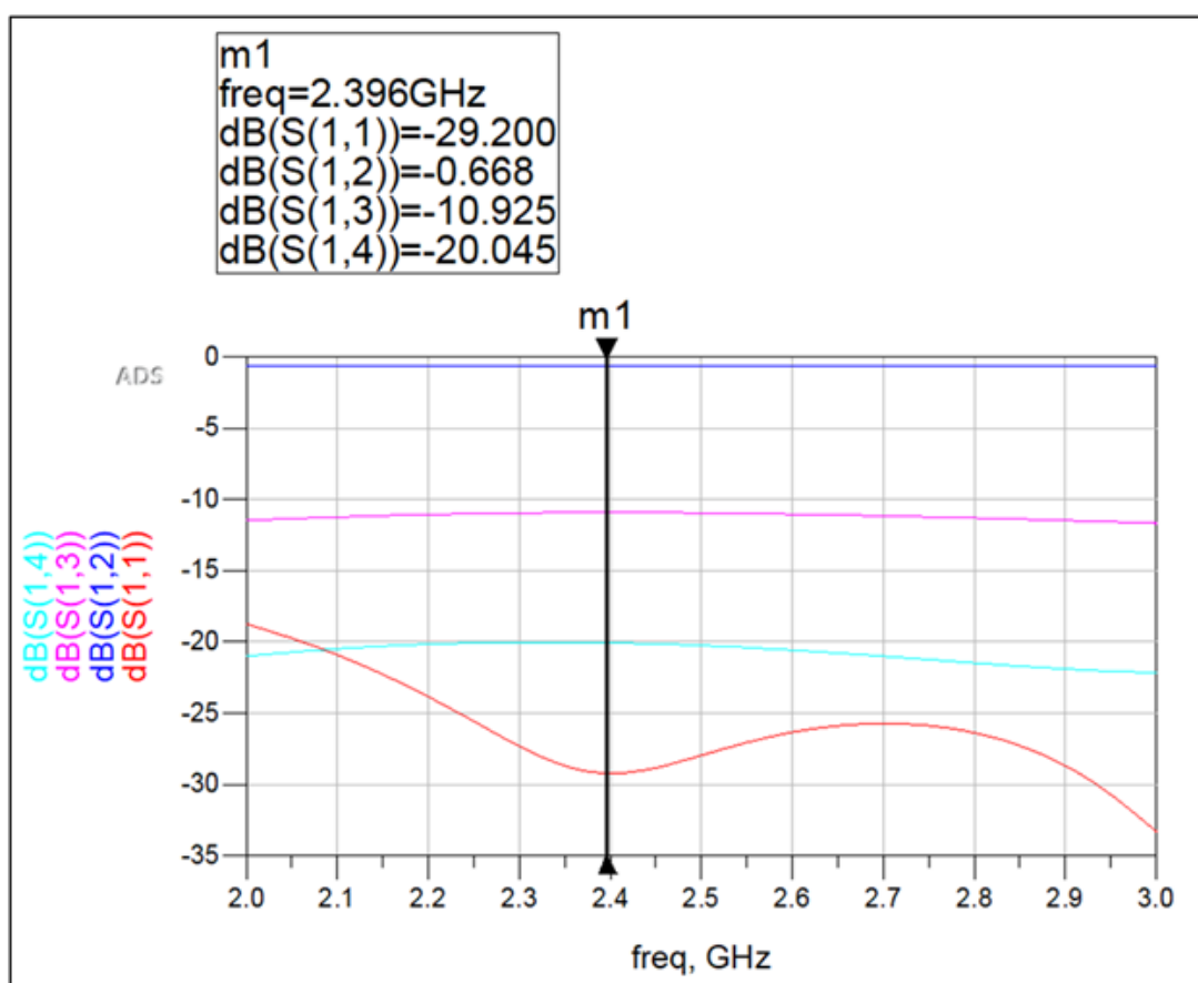
Hình 3.16: Kết quả sau khi chạy mô phỏng layout của Coupled Line Directional Coupler.
