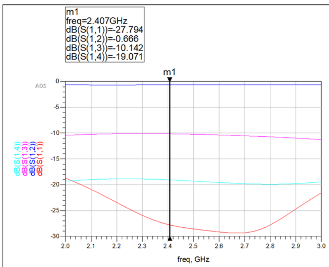
Hình 3.14: Kết quả mô phỏng.
