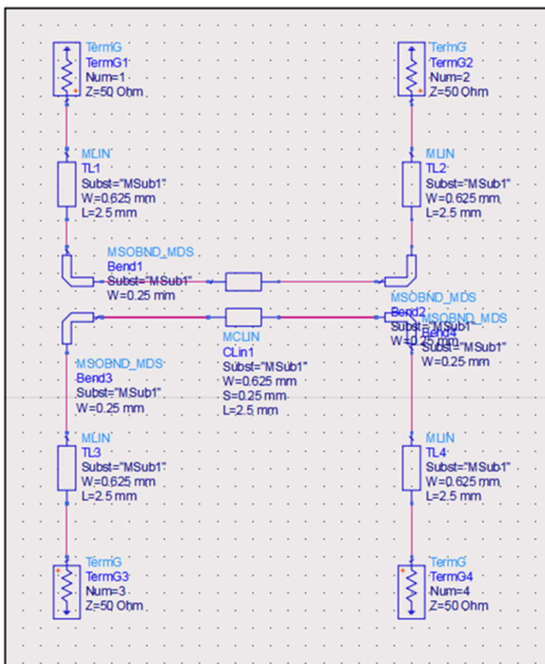
Hình 3.6: Schematic sơ bộ của Coupled Line Directional Coupler.
