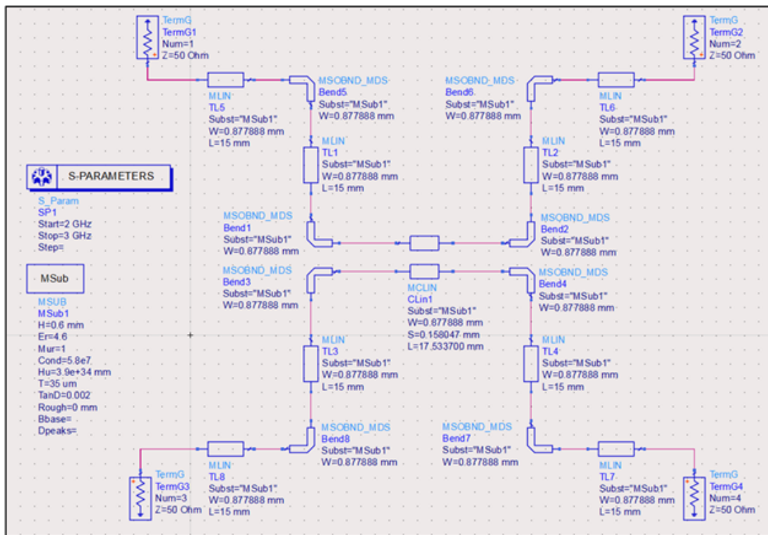
Hình 3.13: Schematic sau khi đã nhập thông số kích thước của microstrip.
