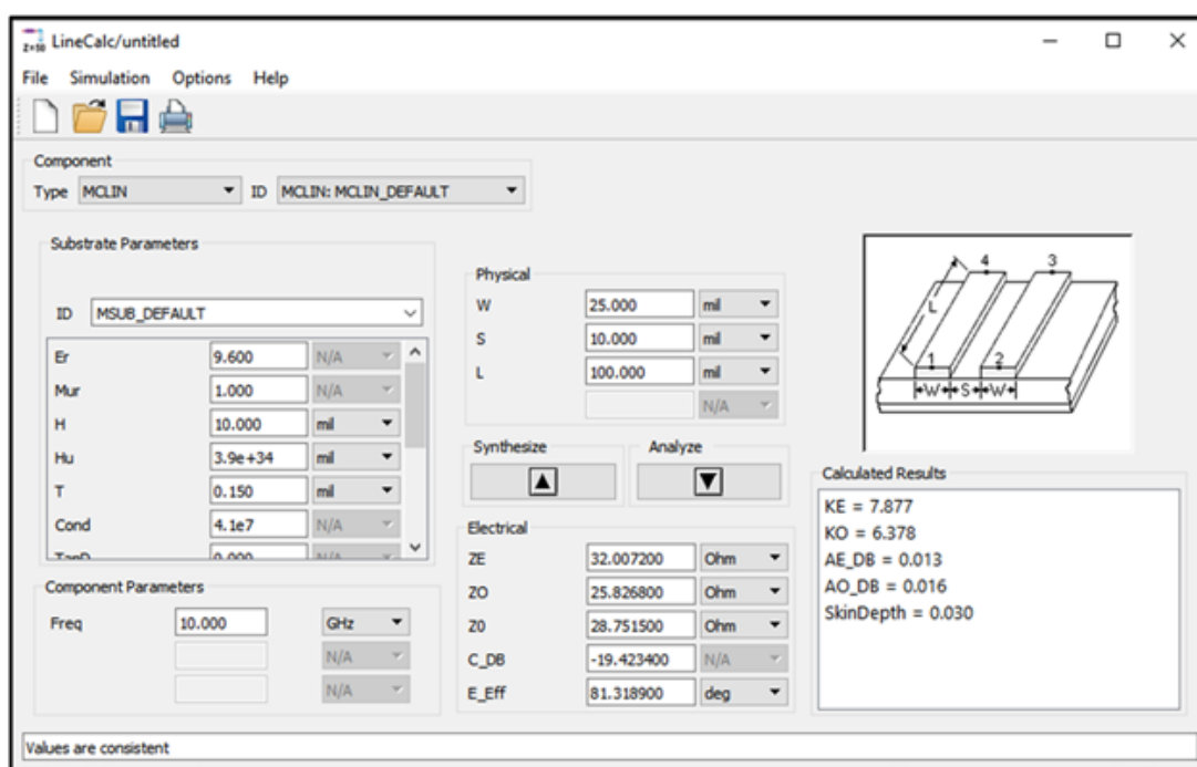
Hình 3.7: Giao diện của LineCalc.
