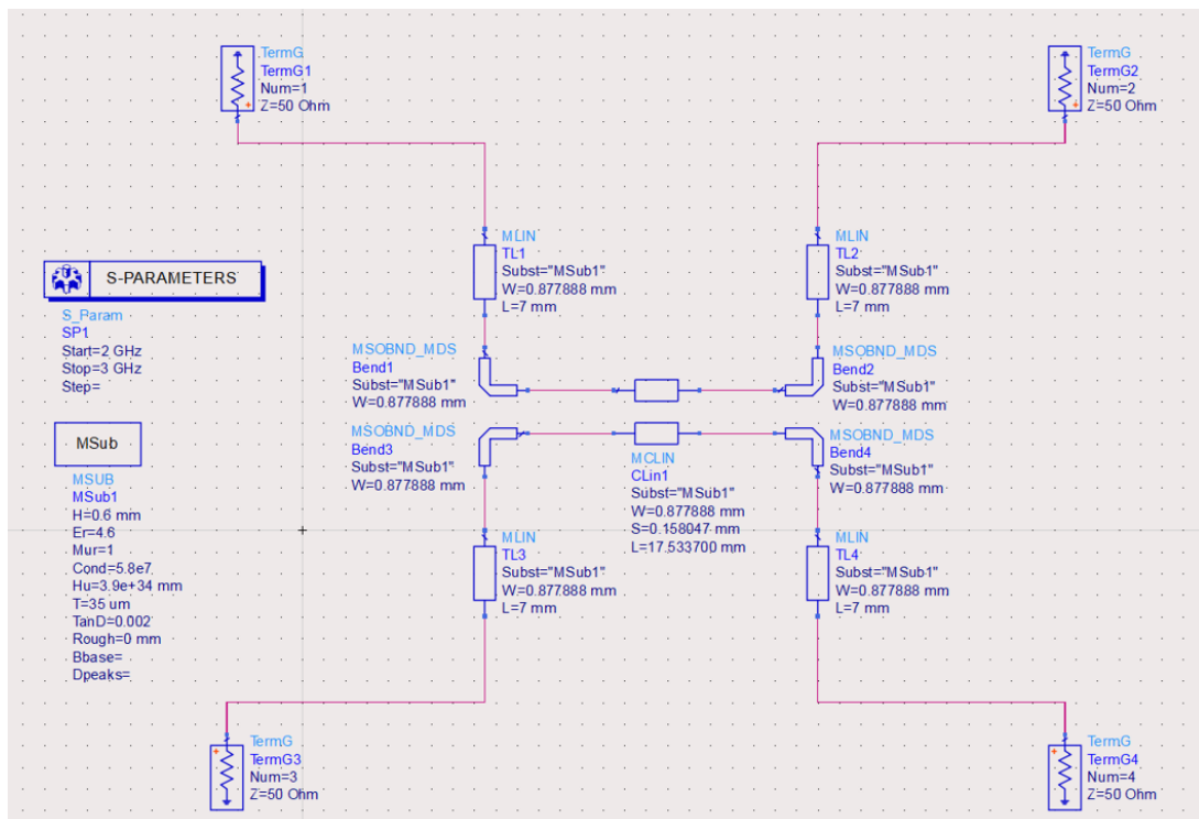
Hình 3.14: Schematic sau khi đã nhập thông số kích thước của microstrip.
