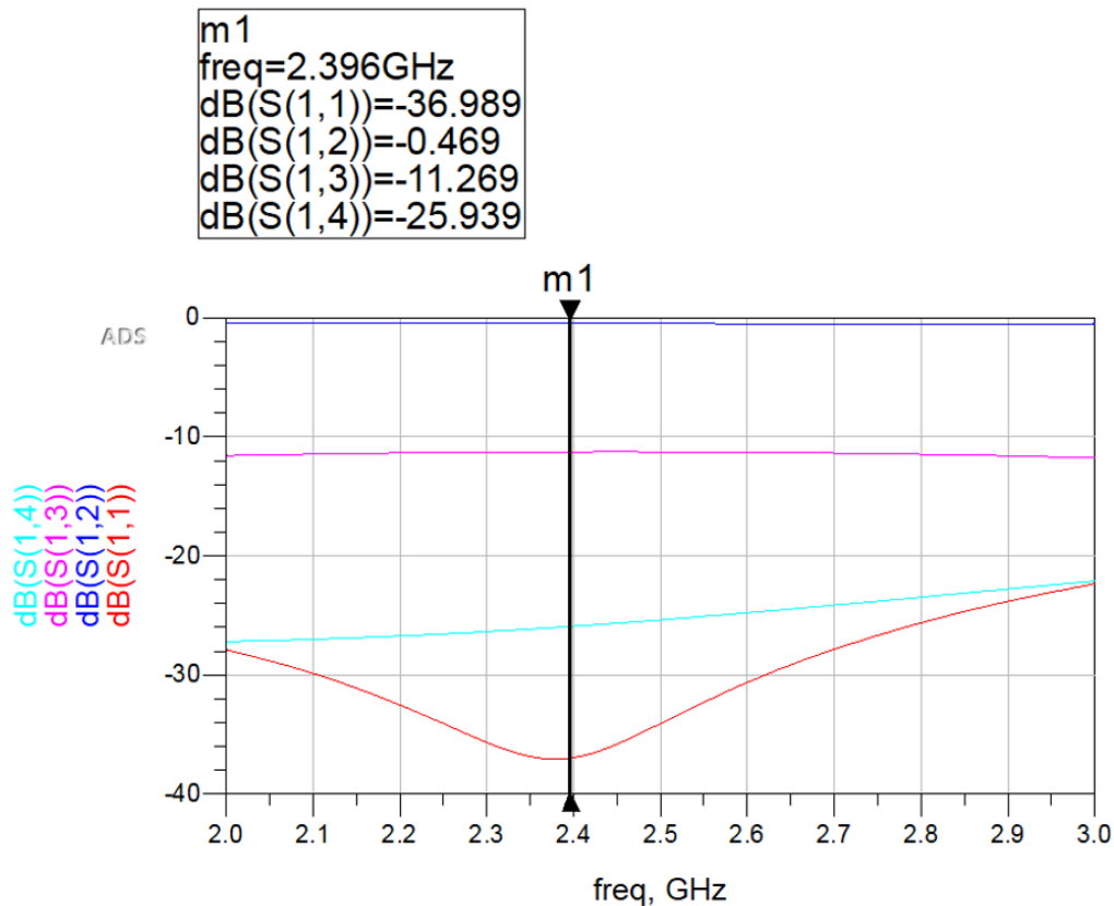
Hình 3.17: Kết quả sau khi chạy mô phỏng layout của Coupled Line Directional Coupler.
