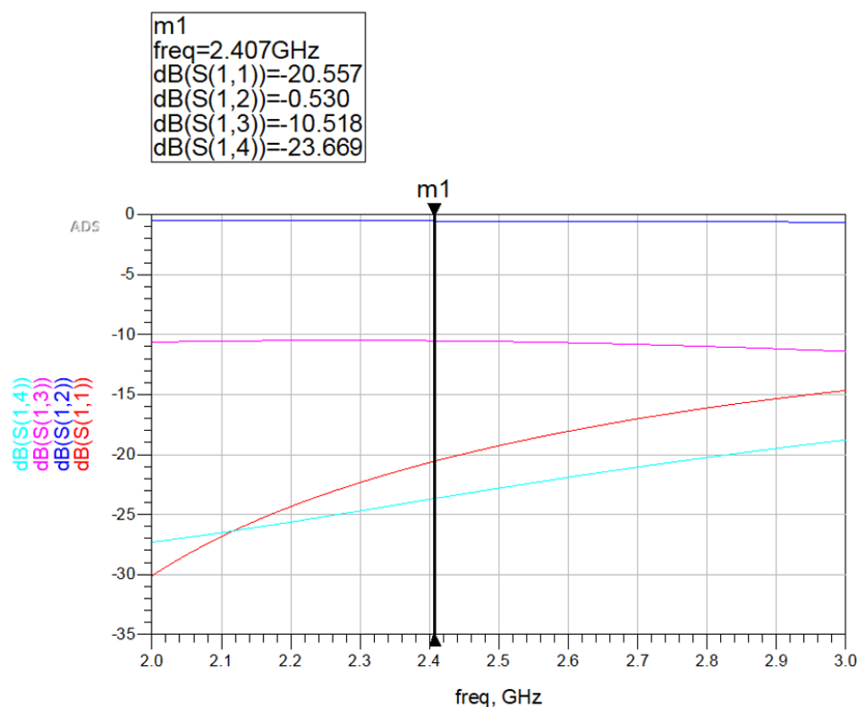
Hình 3.15: Kết quả mô phỏng.
