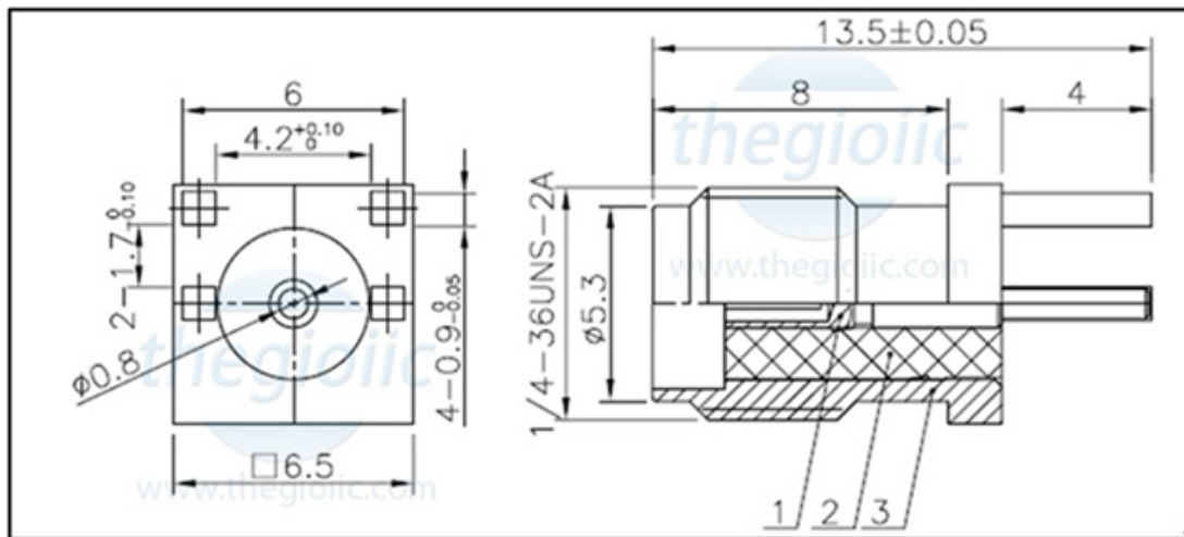
Hình 3.13: Các thông số kích thước của đầu SMA cái 13.5 mm.
