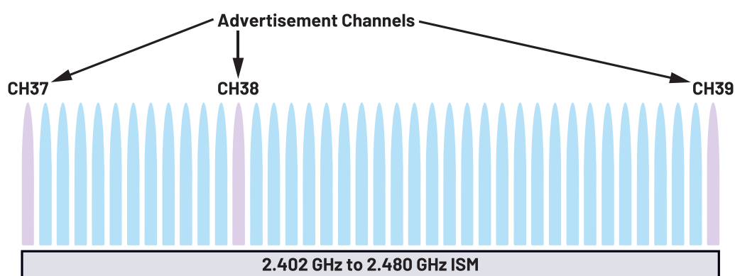
Hình 2.1: BLE channels.
