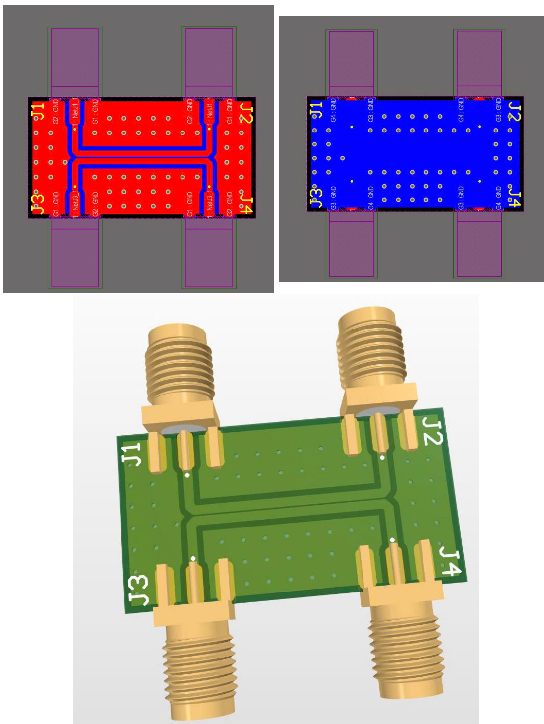
Hình 4.3: Hình ảnh 3D của mạch của Directional Coupler.
