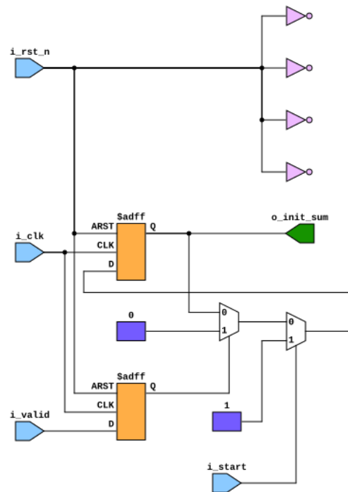
Hình 3: Bộ phát hiện tính hiệu bất đầu.
