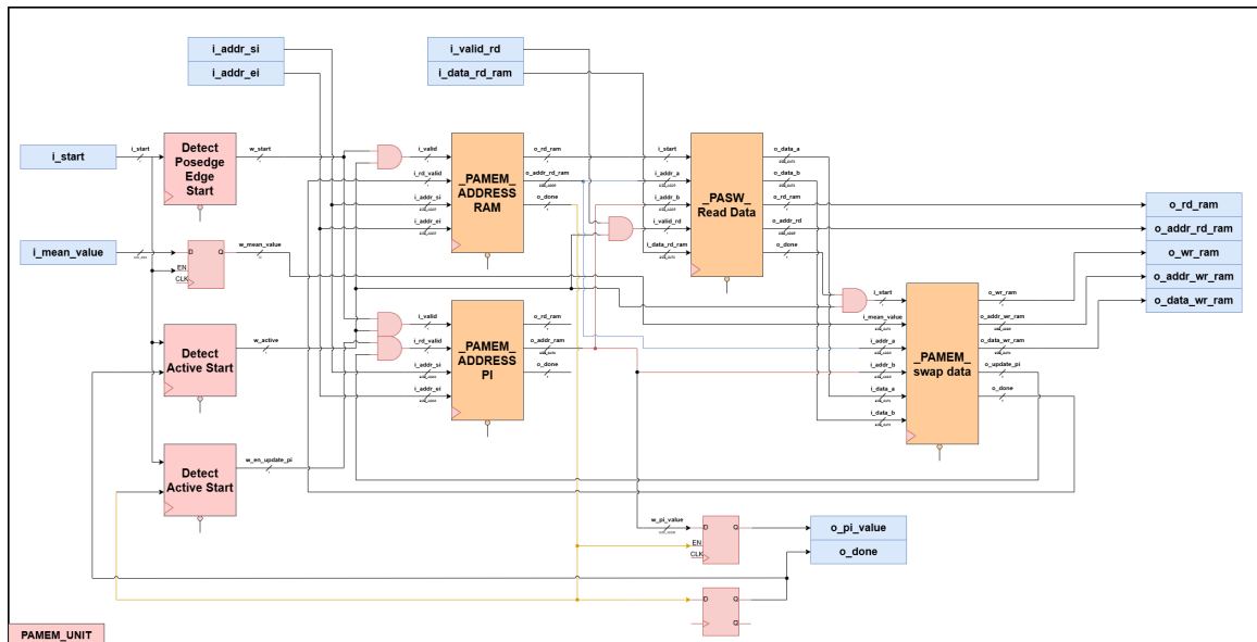
Hình 13: Bộ thực hiện phân hoạch lại mảng dữ liệu
