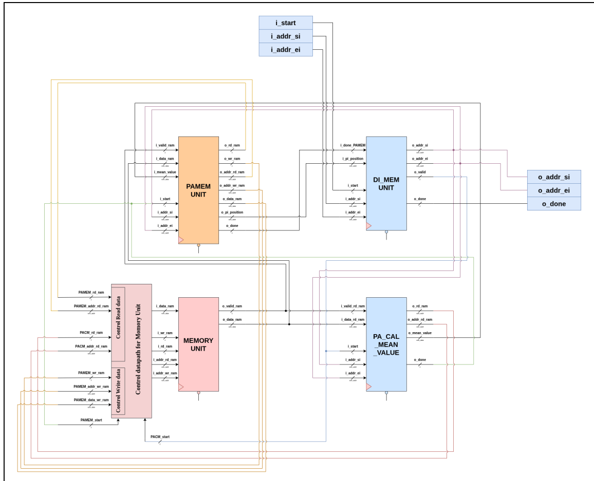
Hình 5: Tổng quan thiết kế của bộ.
