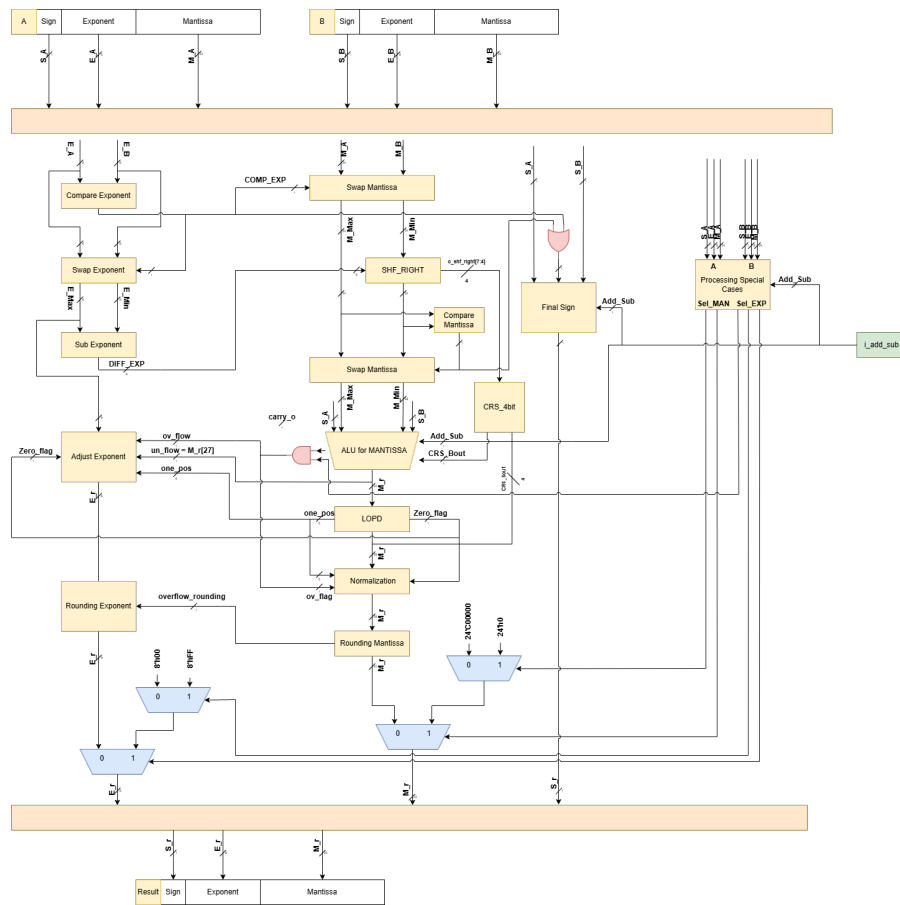
Hình 9: Bộ thực hiện 2 số Floating Point 32-bit.
