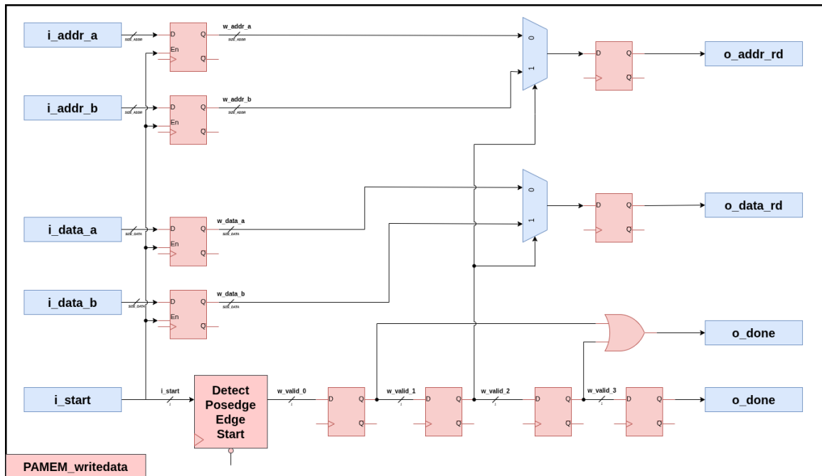
Hình 17: Bộ thực hiện ghi dữ liệu vào lại bộ nhớ.
