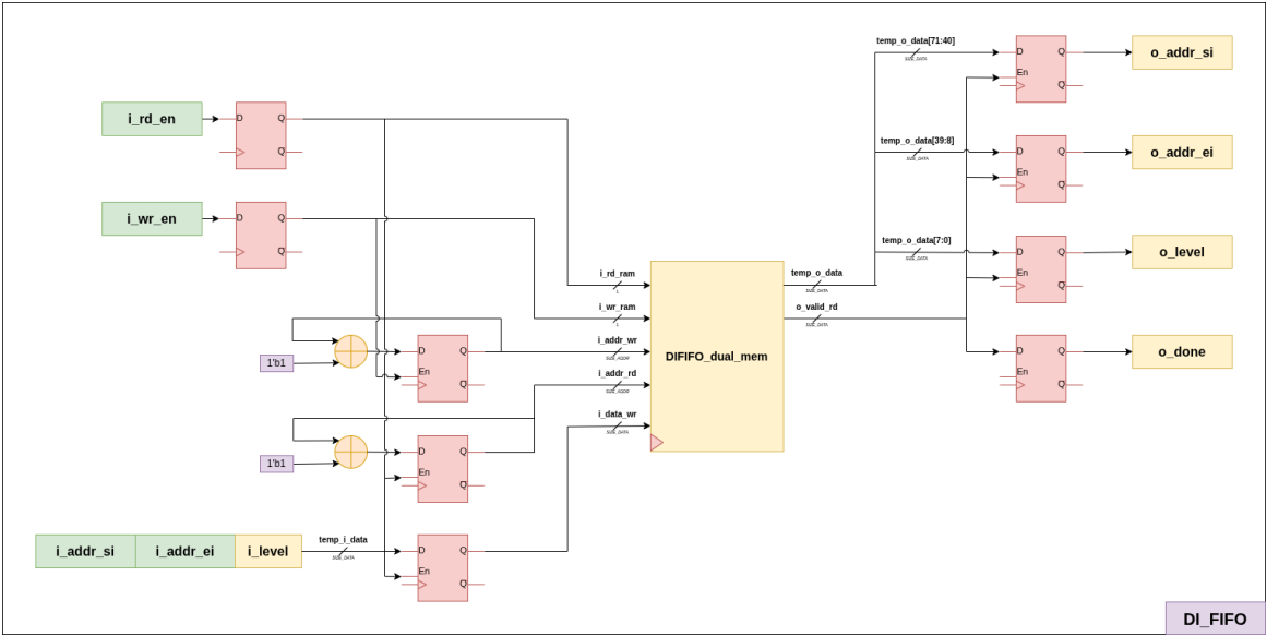
Hình 20: Phần tử nhớ các dữ liệu địa chỉ phân hoạch.
