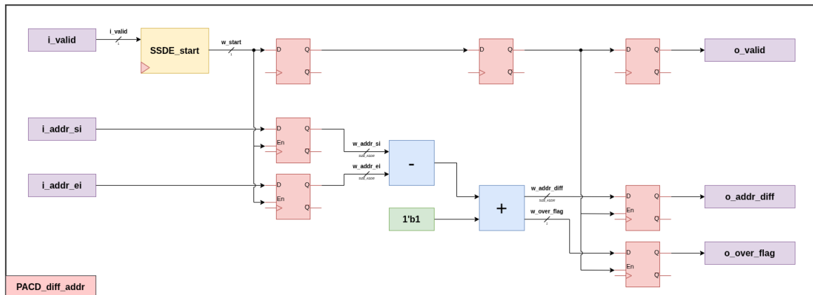
Hình 11: Bộ tính giá trị khoảng cách giữa hai addr_si đến addr_ei .
