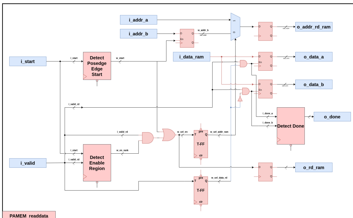
Hình 14: bộ đọc dữ liệu cho hàm.
