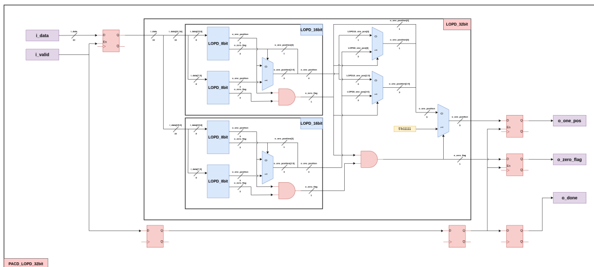
Hình 12: Bộ phát hiện bit 1 của dữ liệu.
