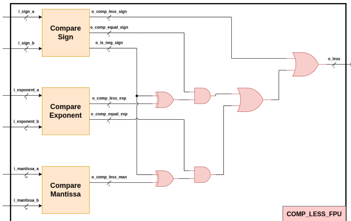
Hình 16: Bộ so sánh Floating Point 32-bit.
