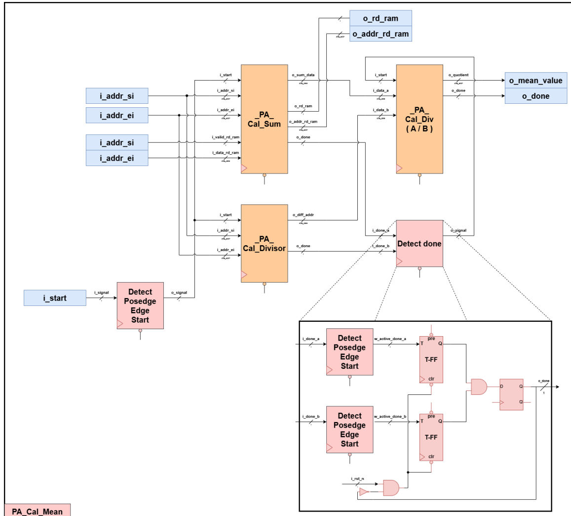
Hình 6: Bộ tính giá trị trung bình của mảng.
