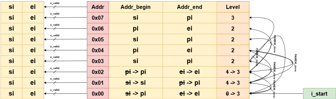
Hình 21: Nguyên tắc hoạt động của bộ điều khiển phân hoạch địa chỉ.
