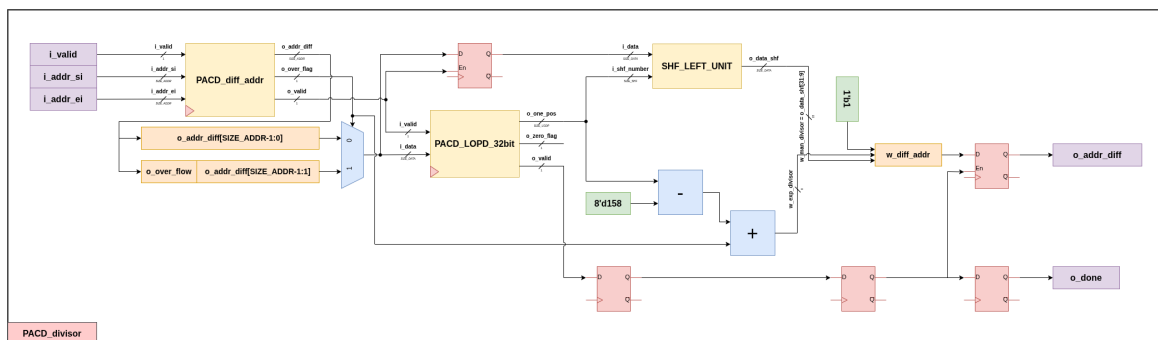
Hình 10: Bộ tính giá trị khoảng cách từ addr_si đến addr_ei .
