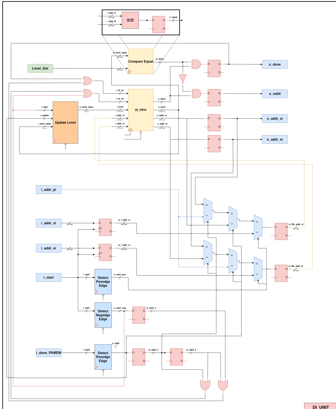
Hình 19: Bộ điều khiển chính trong việc kiểm soát địa chỉ phân hoạch.
