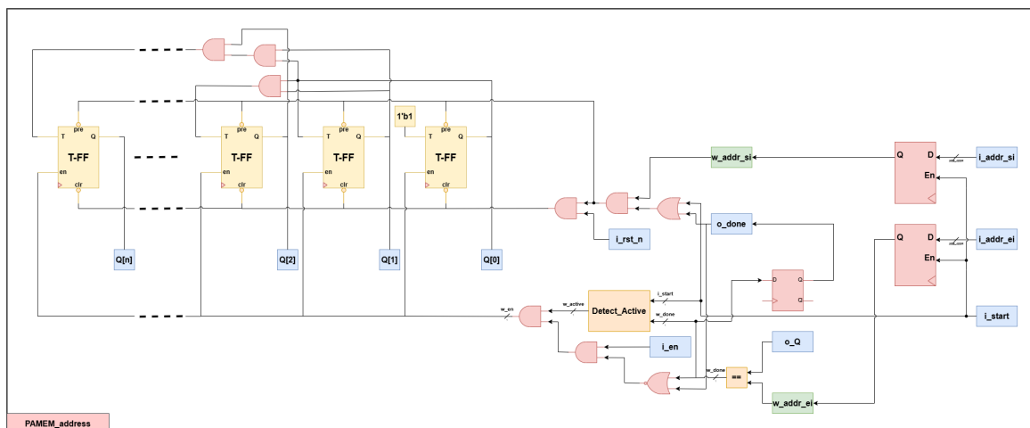
Hình 18: Bộ thực hiện điều khiển hai con trỏ địa chỉ.
