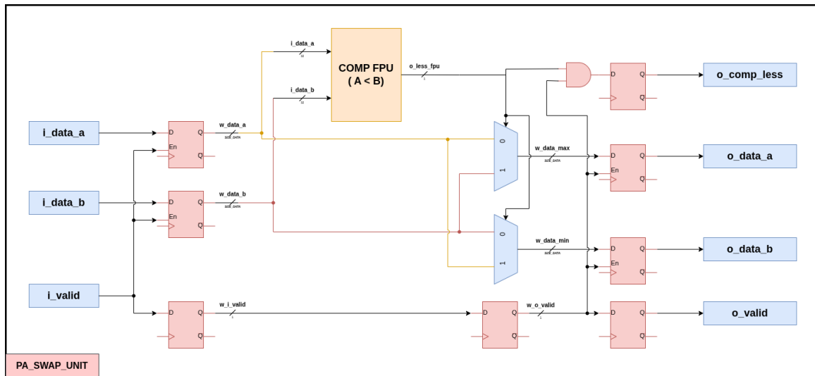
Hình 15: Bộ thực hiện và hoán vị vị trí cho dữ liệu ghi vào bộ nhớ.
