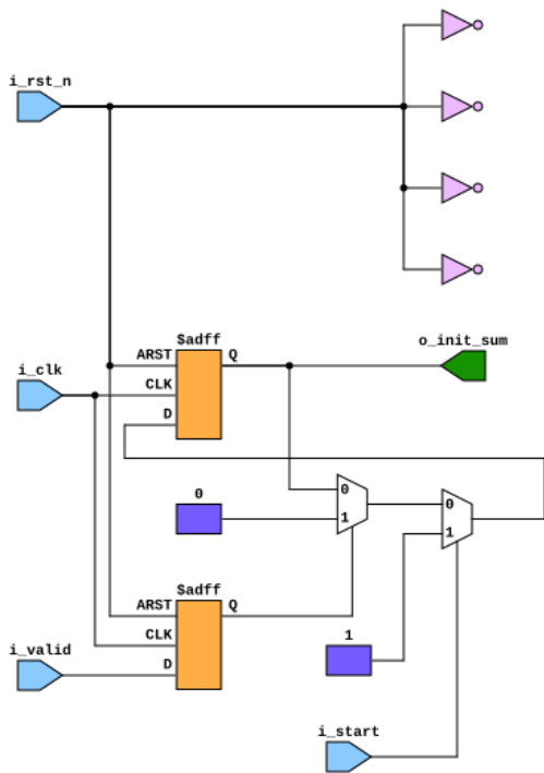
Hình 7: Bộ phát hiện tín hiệu bắt đầu.
