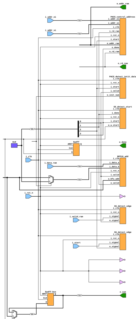
Hình 8: Bộ tính cộng số thực (BFP16_add).
