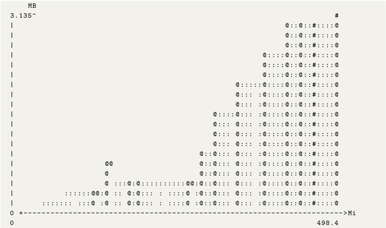
Listing 2: Kết quả kiểm chứng khi chạy với N = 2^{17} .
