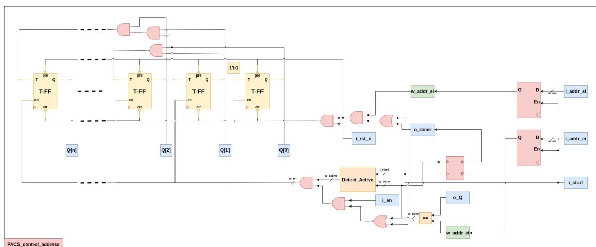
Hình 8: Bộ tính đọc dữ liệu trong mảng.
