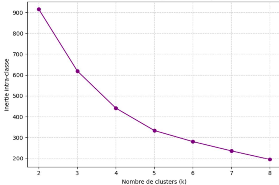
Méthode du coude (Elbow Method)
