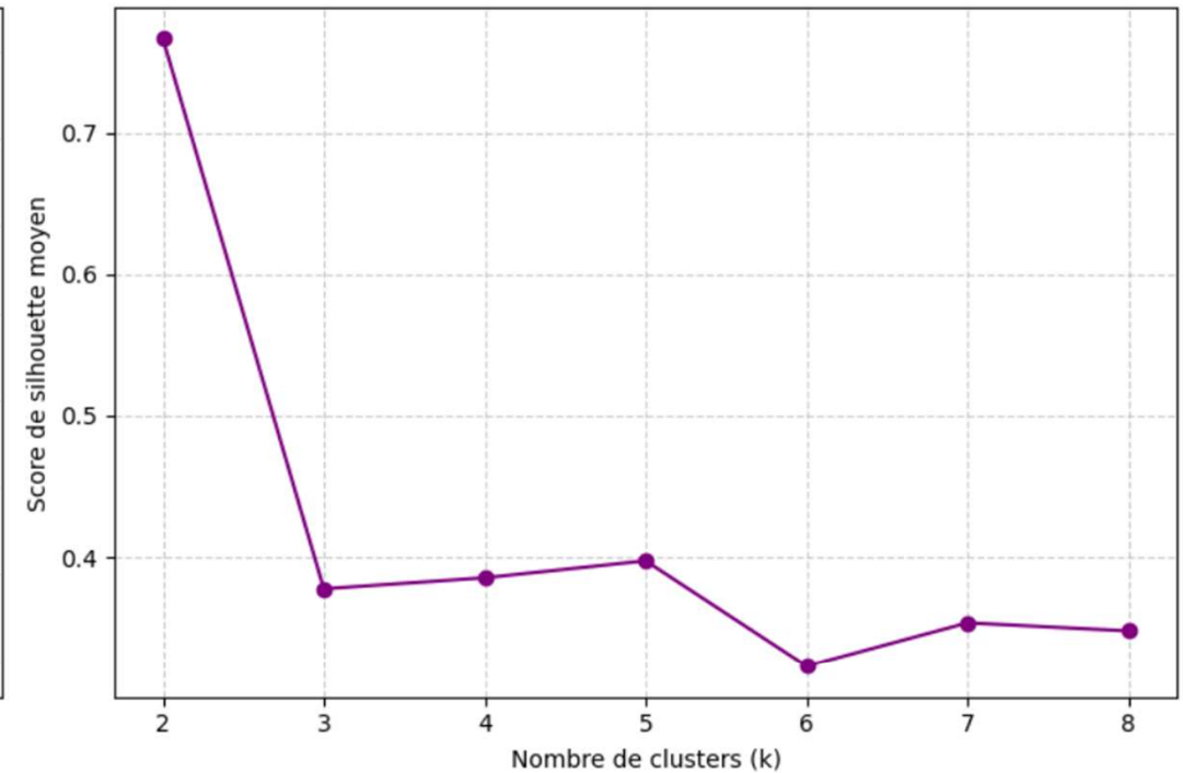
Score de silhouette
