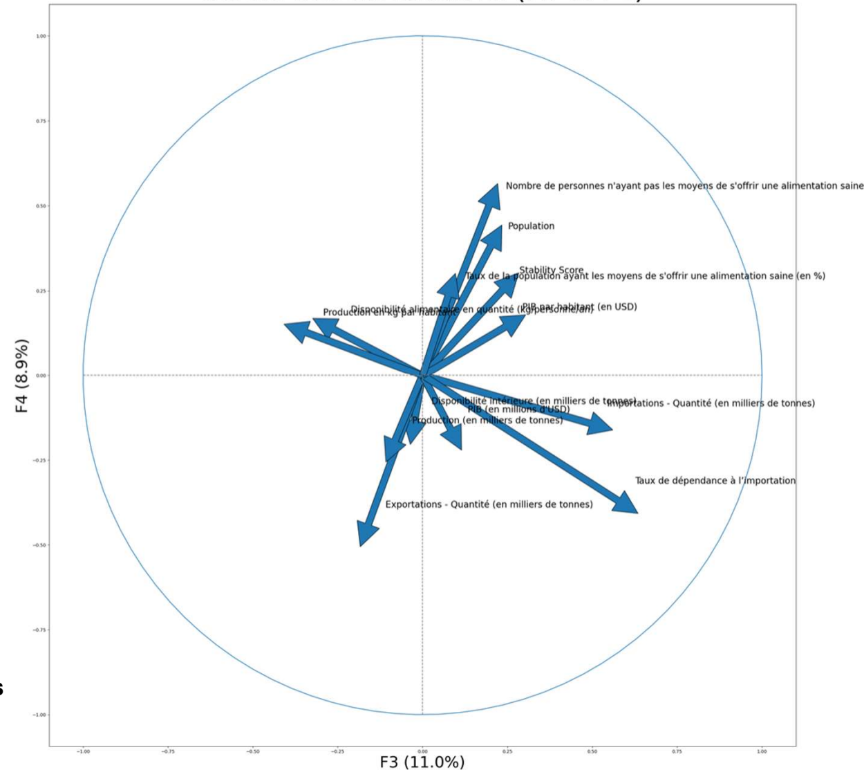
Cercle des corrélations (F3 et F4)
