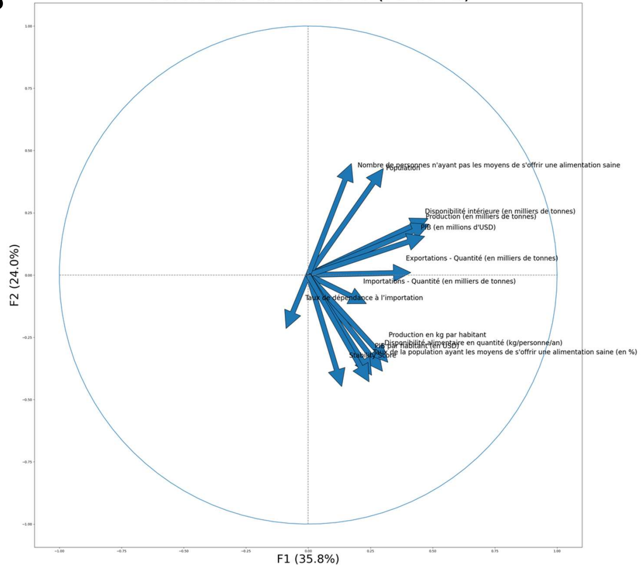
Cercle des corrélations (F1 et F2)
