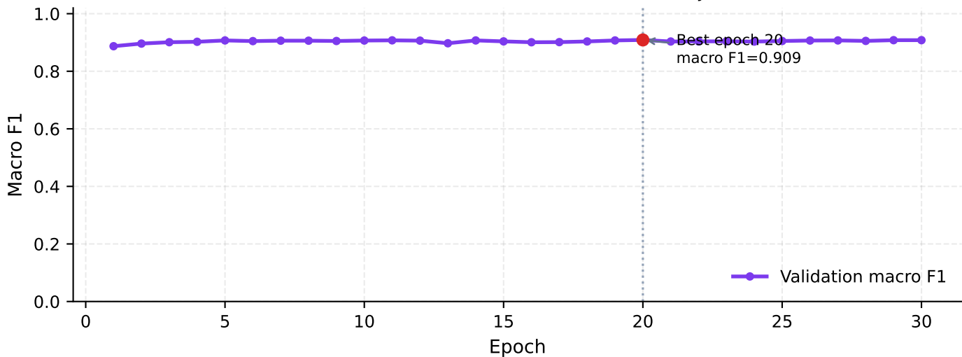
(b) Validation macro F1 (Validation (5 subjects))
