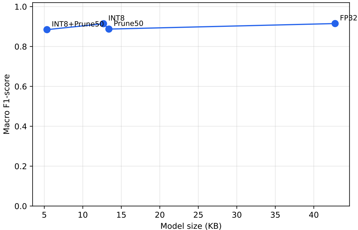
Pareto: macro F1 vs. model size
