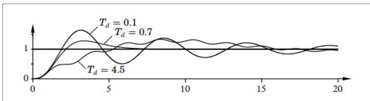
Figure 6: Simularea unui sistem în buclă închisă folosind componentele proporțională, integrală și derivativă. Funcția de transfer a procesului este G(s)=(s+1)^{-3} . Graficul arată valoarea dorită (setpoint) care este egală cu 1 și ieșirea buclei pentru K_p = 3 , K_i = 3 și diferite valori pentru K_d unde K_d = K_p \times T_d (sursa: [9])
