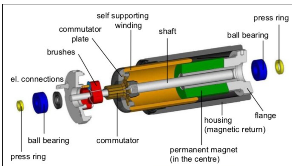
Figure 3: Motor cu perii de tip coreless(sursa: [8])
