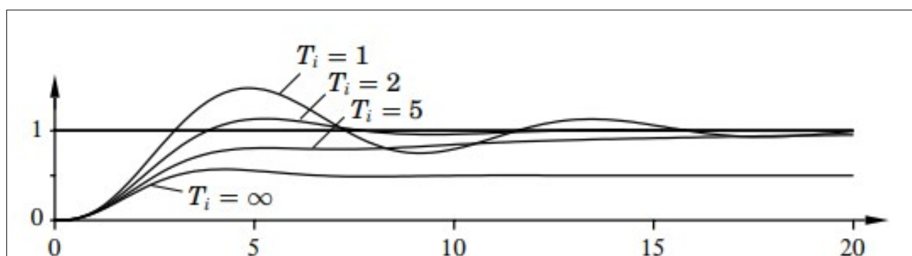
Figure 5: Simularea unui sistem în buclă închisă folosind componenta proporțională și cea integrală. Funcția de transfer a procesului este G(s) = (s+1)^{-3} . Graficul arată valoarea dorită (setpoint) care este egală cu 1 și ieșirea buclei pentru K_p = 1 și pentru diferite valori ale K_i unde K_i = K_p/T_i . (sursa: [9])
