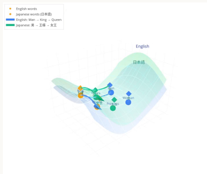
Animation: Japanische & englische Wort-Mannigfaltigkeiten, verbunden durch Translation + Rotation
