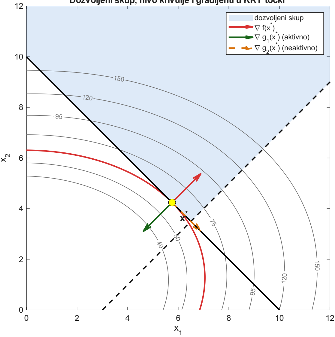
Dozvoljeni skup, nivo krivulje i gradijenti u KKT točki
