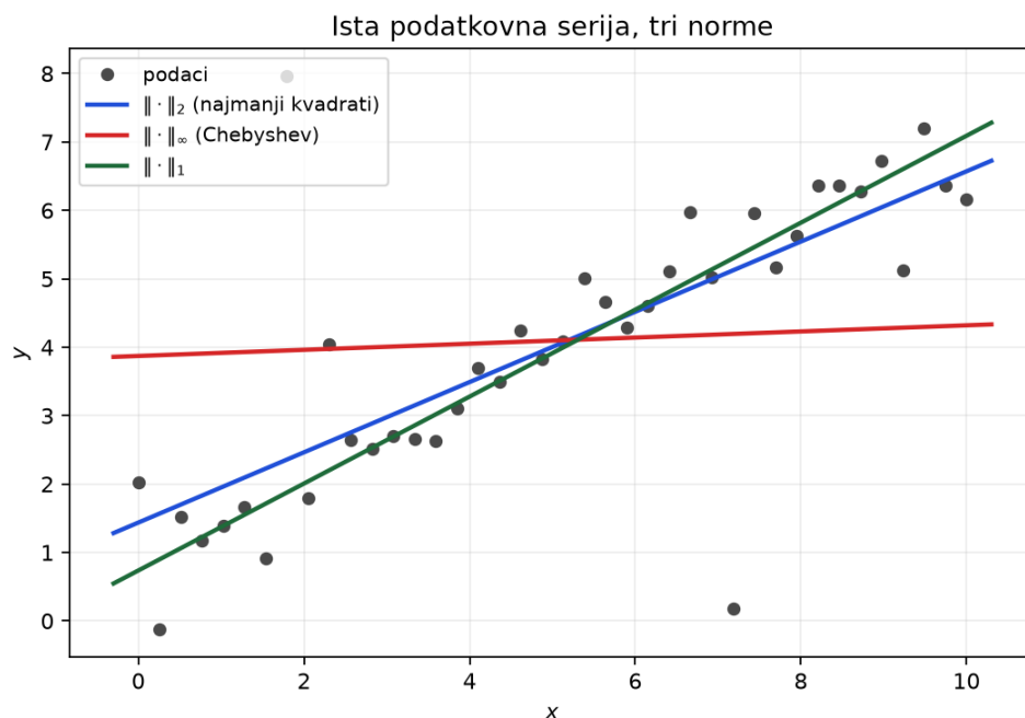
Slika 5.3: Ista podatkovna serija (s dvije namjerno ubačene stršeće vrijednosti), aproksimirana pravcem u tri norme. \infty -norma pokušava zadovoljiti i najgoru točku, pa se pravac potpuno izobliči; 1-norma je najotpornija.
