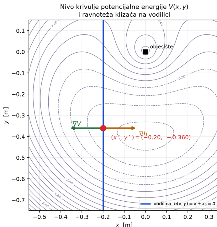
Slika 3.4: Rekonstrukcija konturnih grafova sa slajdova 66--67: nivo krivulje potencijalne energije V(x, y) , vodilica x = -x_0 (plavo) i ravnotežni položaj u kojem su \nabla V i \nabla h kolinearni.
