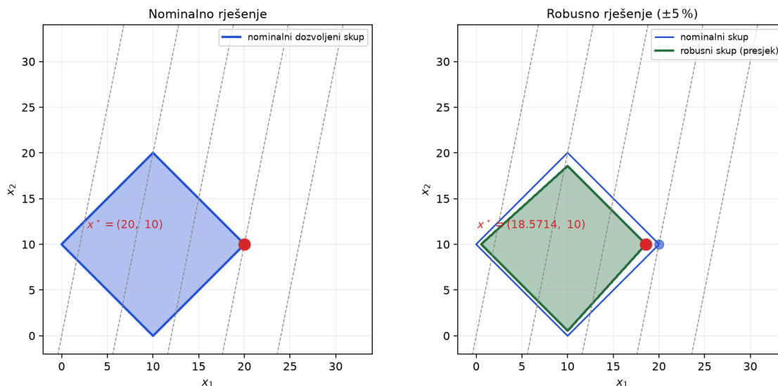
Slika 8.1: Lijevo: nominalni problem, optimum u vrhu (20, 10). Desno: robustni skup (presjek dozvoljenih skupova preko svih perturbacija) je manji od nominalnog, pa se optimum pomiče u (18,5714; 10). Isprekidane linije su nivo krivulje funkcije cilja.
