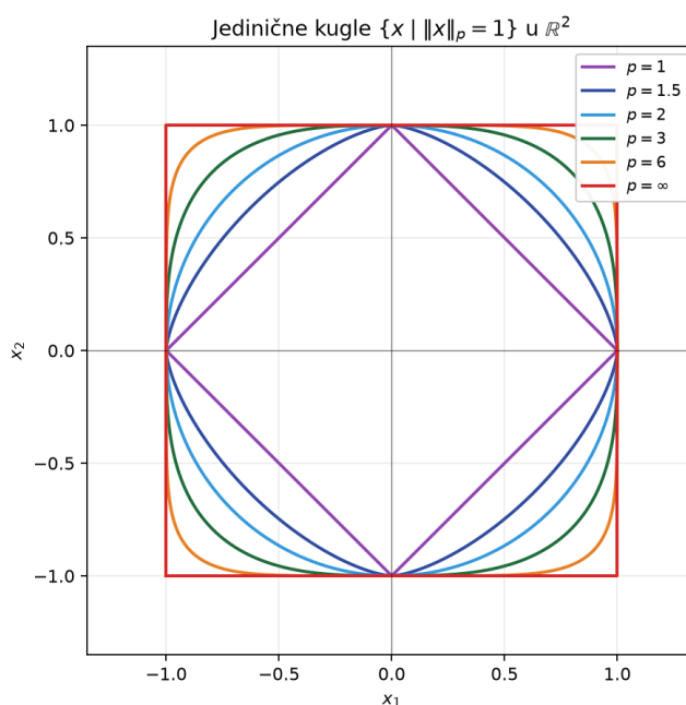
Slika 2.4: Jedinične kugle p -normi u \mathbb{R}^2 : romb ( p = 1 ), kružnica ( p = 2 ) i kvadrat ( p = \infty ), s međuslučajevima.
