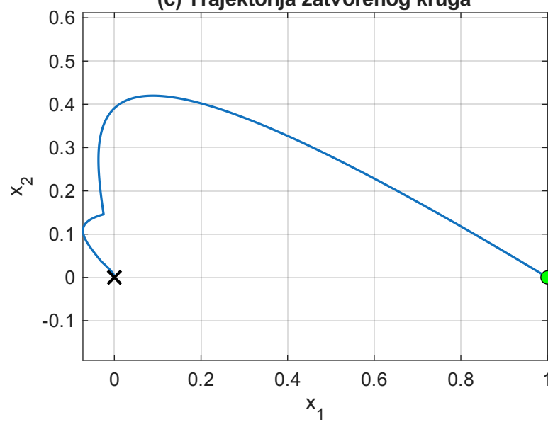
(c) Trajektorija zatvorenog kruga
