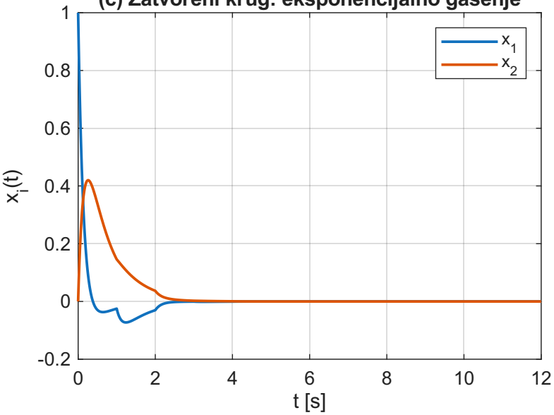
(c) Zatvoreni krug: eksponencijalno gasenje
