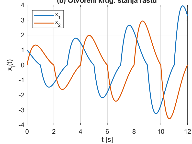
(b) Otvoreni krug: stanja rastu
