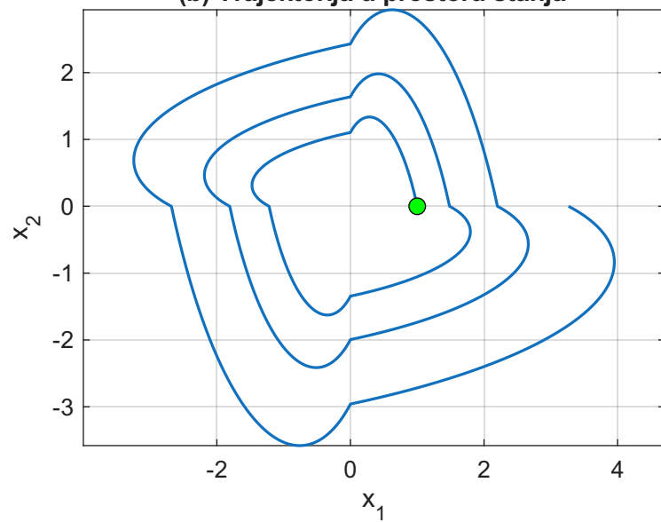
(b) Trajektorija u prostoru stanja
