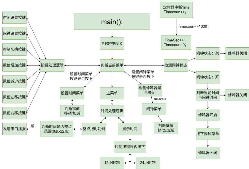
图 4-1 软件整体框架流程图
