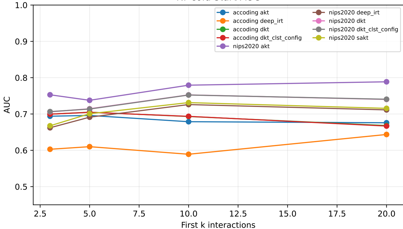
KT cold-start AUC
