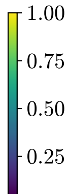
Gradient-SHAP
