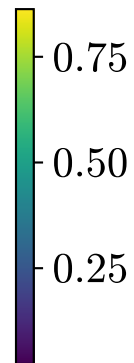
Gradient-SHAP
