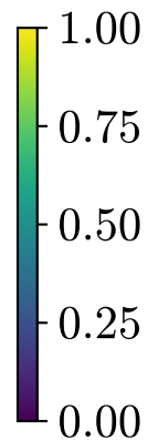
Gradient-SHAP
