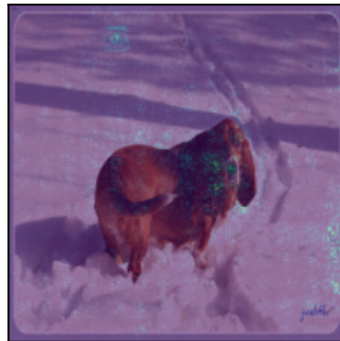
Gradient-SHAP
