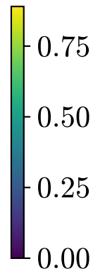
Gradient-SHAP
