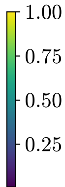
Gradient-SHAP
