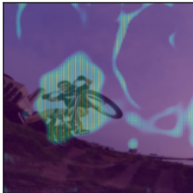
Ours
