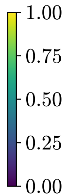
Gradient-SHAP
