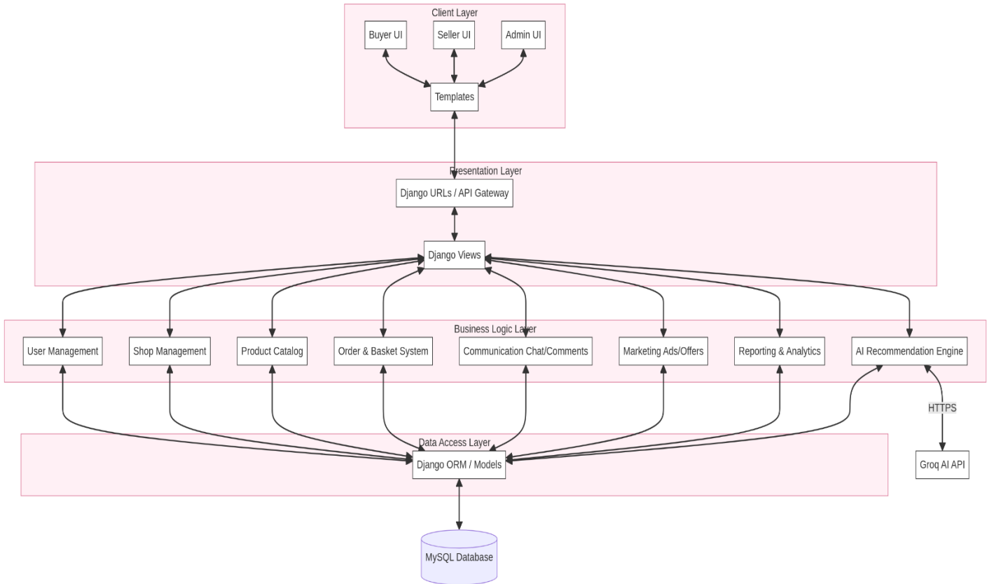
الشكل 82 Component diagram
