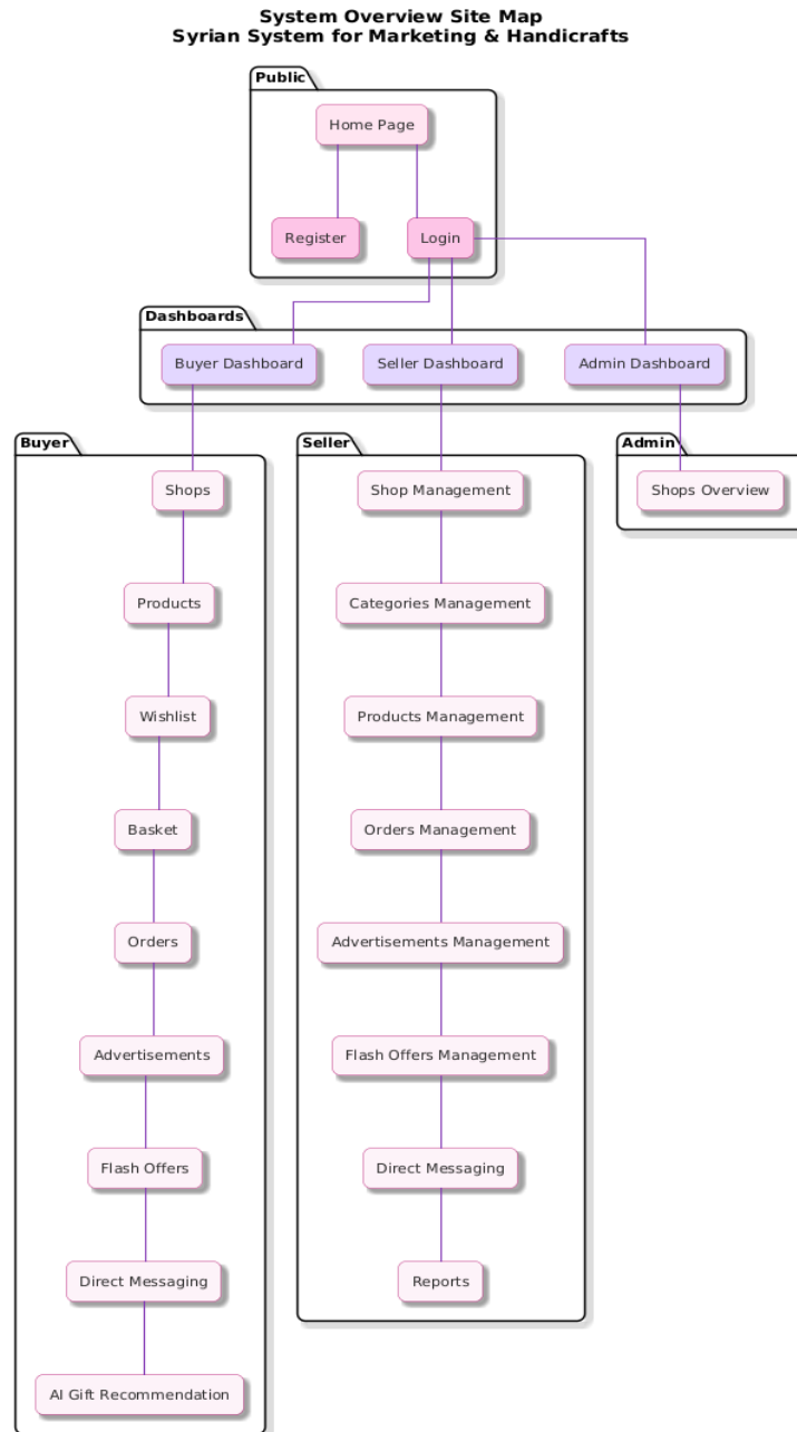
الشكل 83 System Overview Site Map
