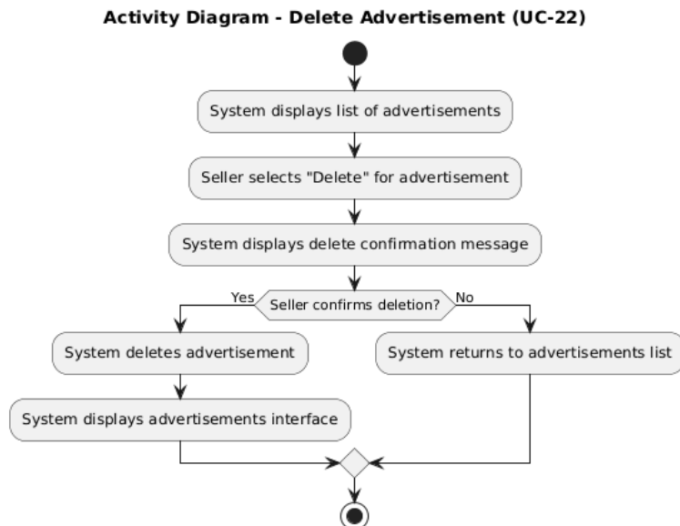
الشكل 26 مخطط نشاط حذف الإعلانات
