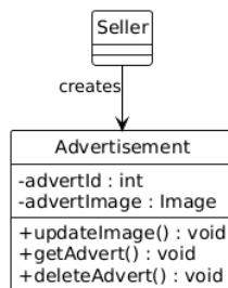
الشكل 74 Advertisements class
