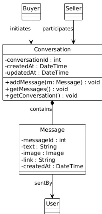
الشكل 77 Messages class
