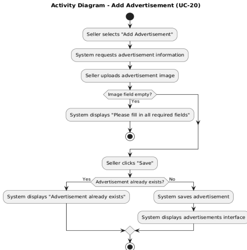
الشكل 24 مخطط نشاط إضافة الإعلانات
