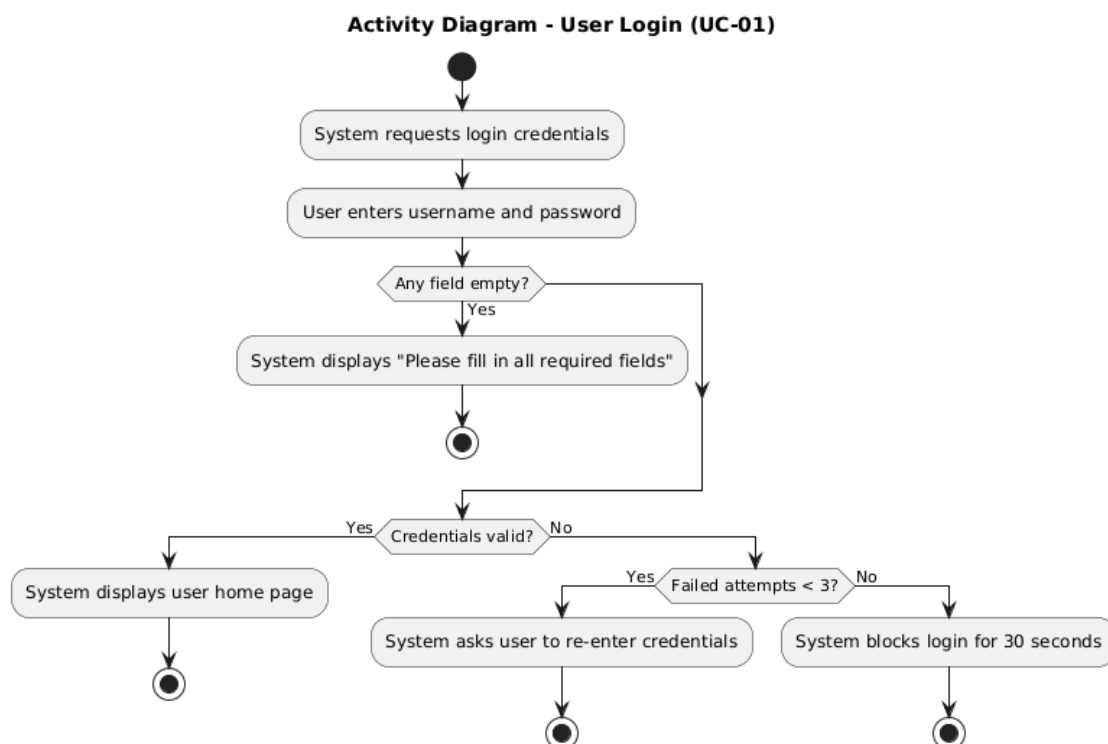
الشكل 5 مخطط نشاط تسجيل الدخول
