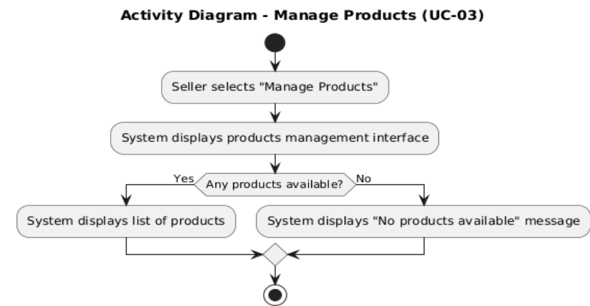
الشكل 7 مخطط نشاط إدارة المنتجات
