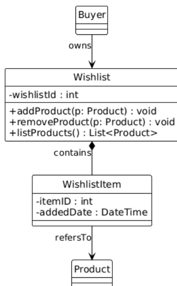
الشكل 76 Wishlist class
