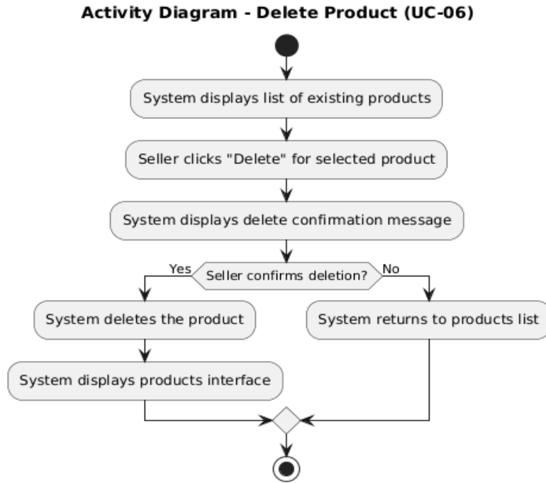
الشكل 10 مخطط نشاط حذف منتج
