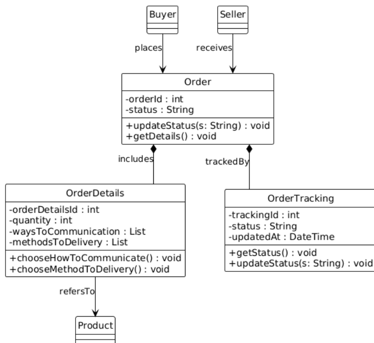
الشكل 72 Orders class
