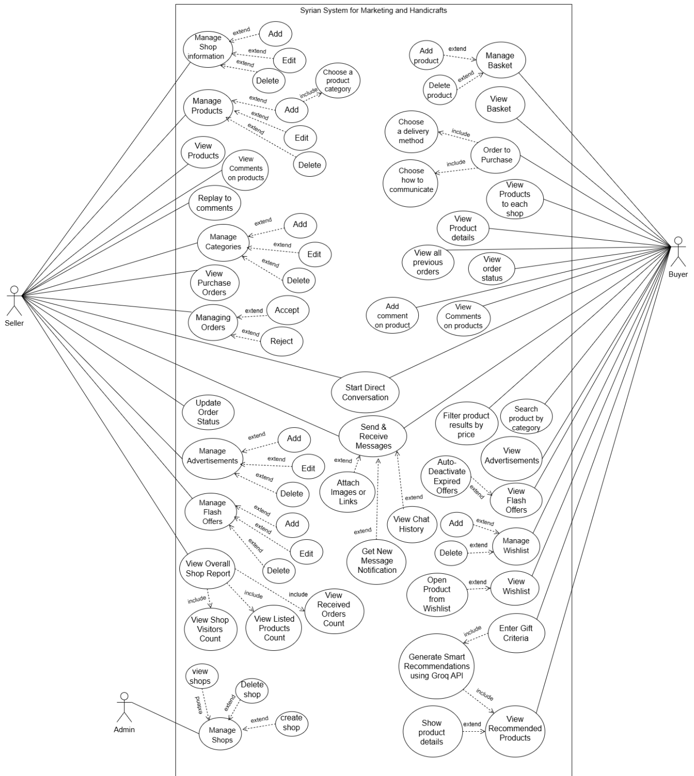
الشكل 4 Low level-use case diagram
