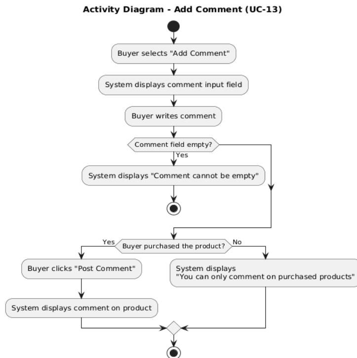
الشكل 17 مخطط نشاط إضافة التعليقات
