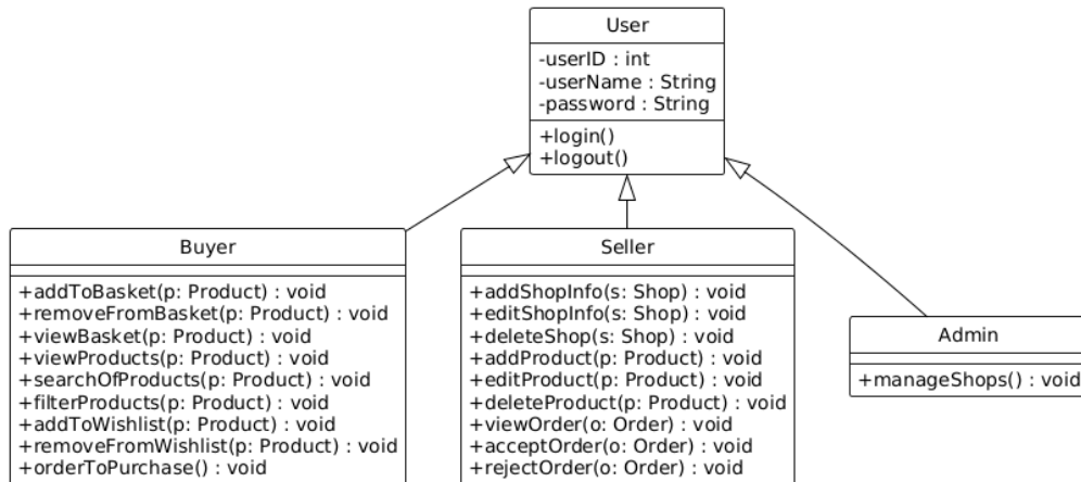
الشكل 69 Users class
