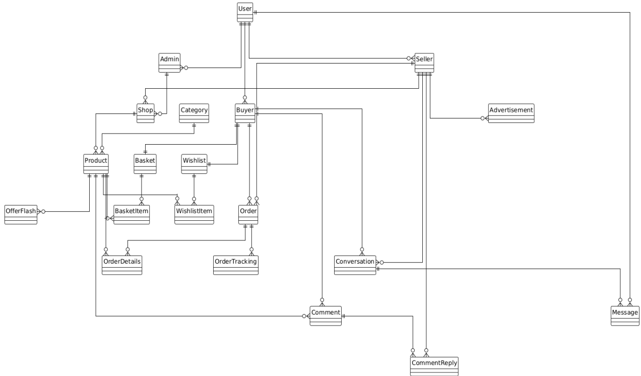
الشكل 79 High level ERD
