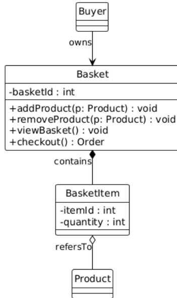
الشكل 71 Basket class
