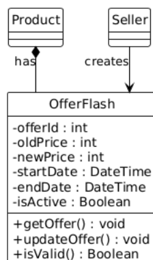
الشكل 75 Offer Flash class
