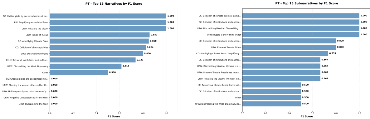
(a) Top narrative F1 scores
