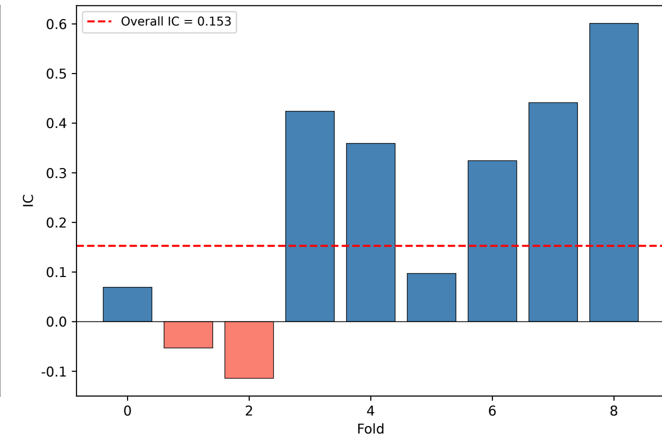
5d: Fold IC
