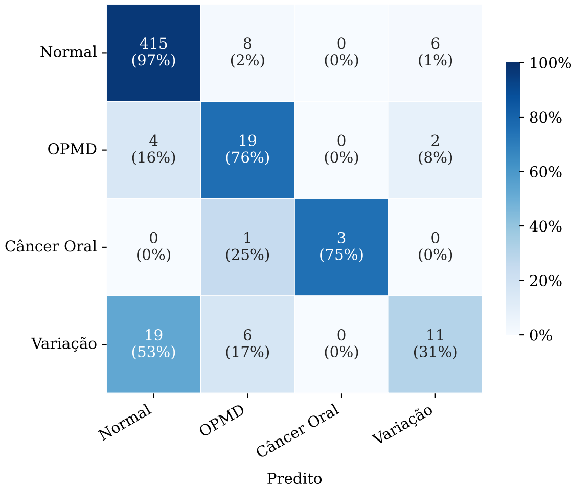
YOLO26m-cls — Classificação Multiclasse
