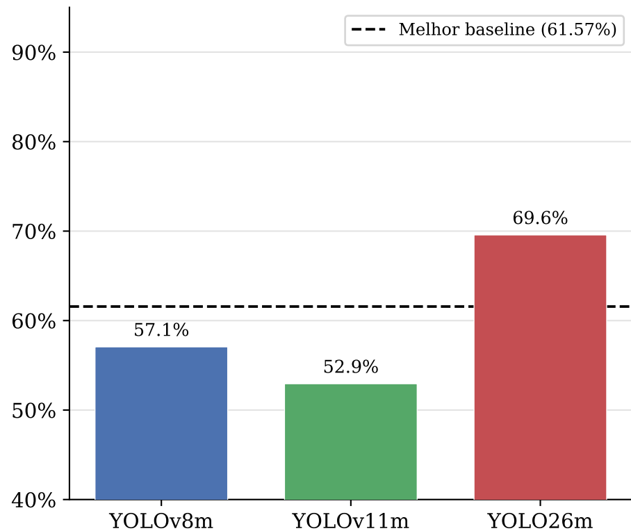
(b) Classificação Multiclasse ( T_2 )
