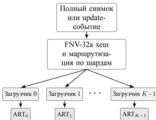
Рисунок 5 – Устройство шардированного ART-хранилища
